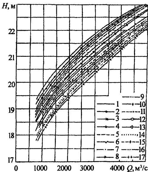
Рис. П1.1. Кривые связи расходов и уровней в нижнем бьефе Новосибирской ГЭС:
