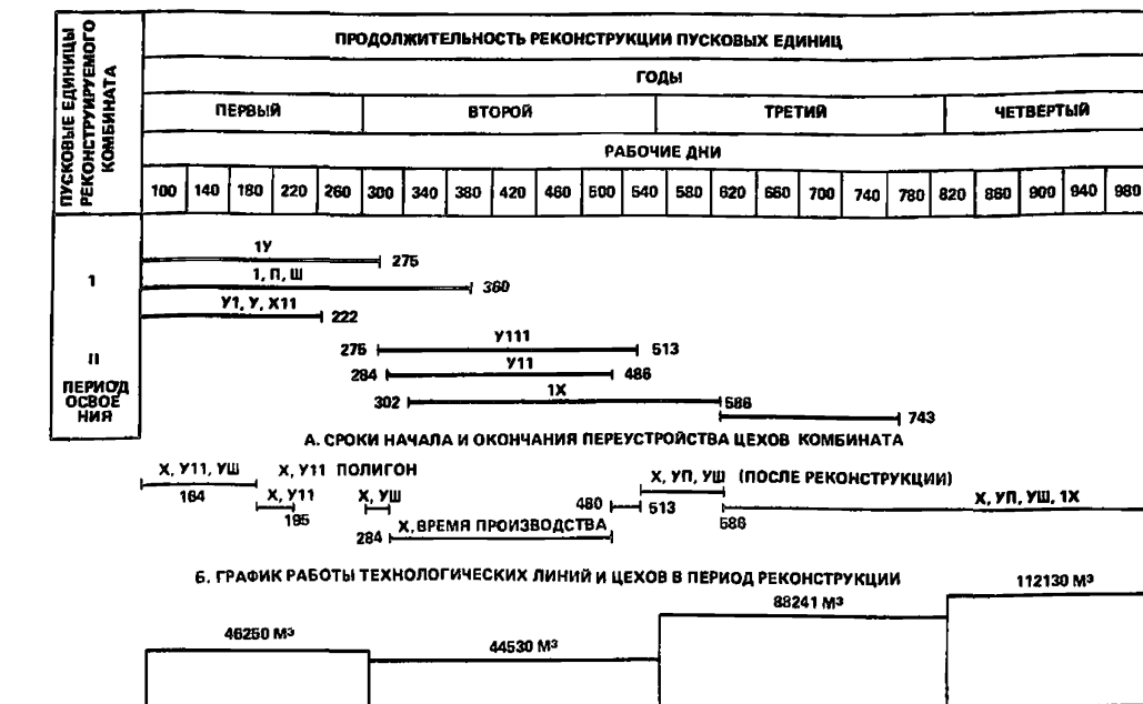
Рис. 1. Производственные мощности домостроительного комбината по годам проведения реконструкции I — Х/II — название цехов; 275 — 513 — сроки начала и окончания реконструкции технологической линии
