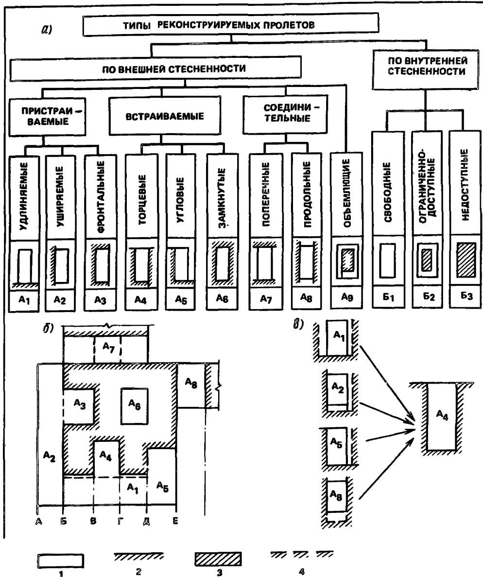
Рис. 3. Типы пролетов, возводимых при реконструкции одноэтажных промзданий
