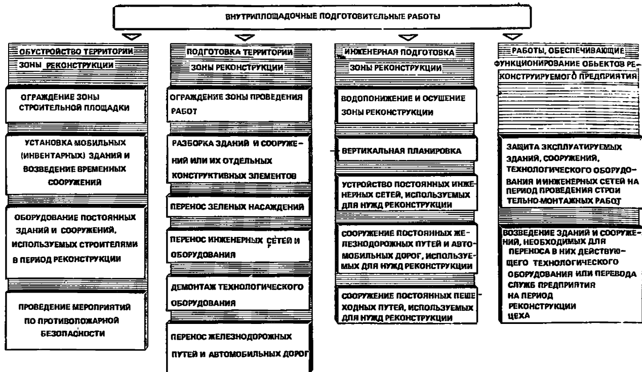
Рис. 5. Схема группировки внутripлощадочных подготовительных работ в зависимости от их функционального назначения, организационной и технологической взаимосвязи
