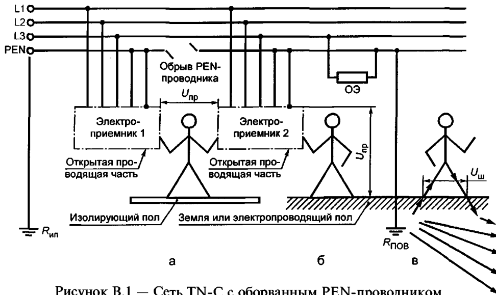
Рисунок В.1 — Сеть TN-C с оборванным PEN-проводником. Уравнивание и выравнивание потенциалов отсутствуют
