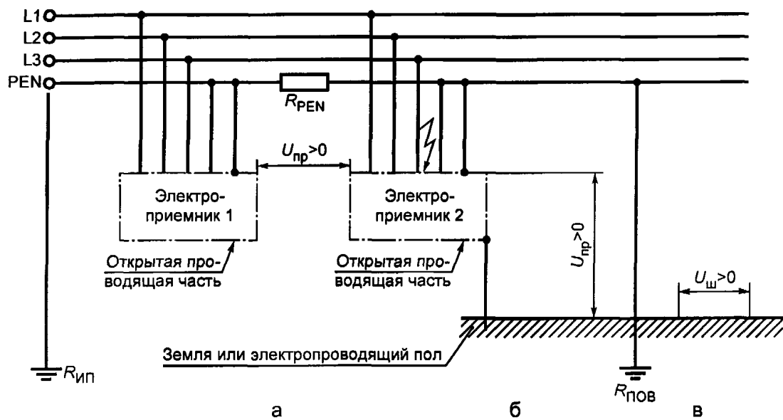
Рисунок В.3 — Сеть TN-C с однофазным замыканием на корпус
