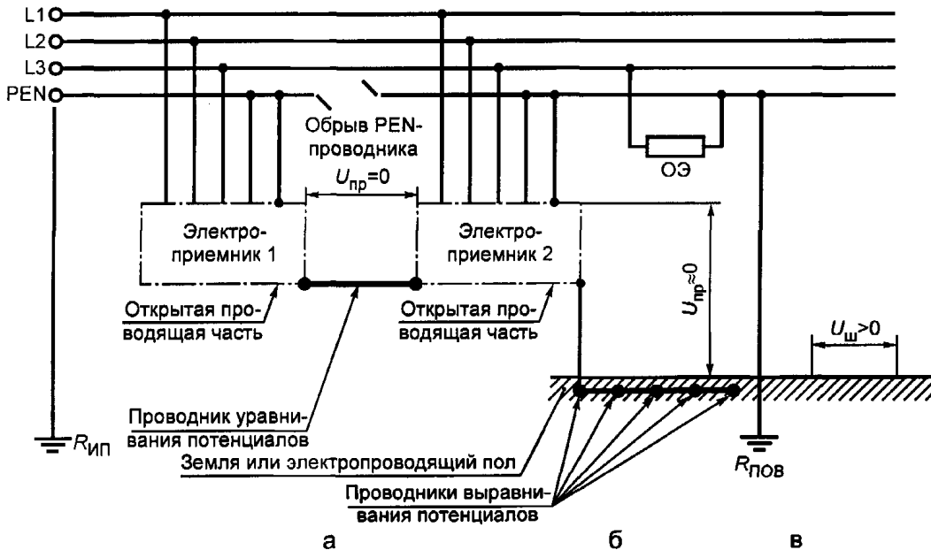
Рисунок В.2 — Сеть TN-C с оборванным PEN-проводником. Имеется уравнивание потенциалов на участке а), выравнивание потенциалов на участке б). На участке в) выравнивание потенциалов отсутствует
