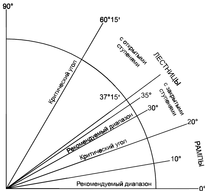
Рисунок 1 — Углы наклона средств доступа к рабочему месту
