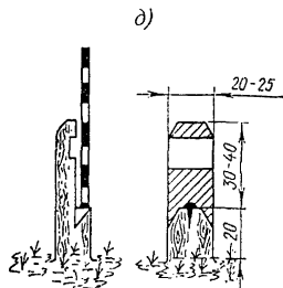
Рис. 4.1. Типы знаков долговременного закрепления пунктов съёмочного обоснования
