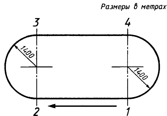
Рисунок А.1 — Испытательный полигон
