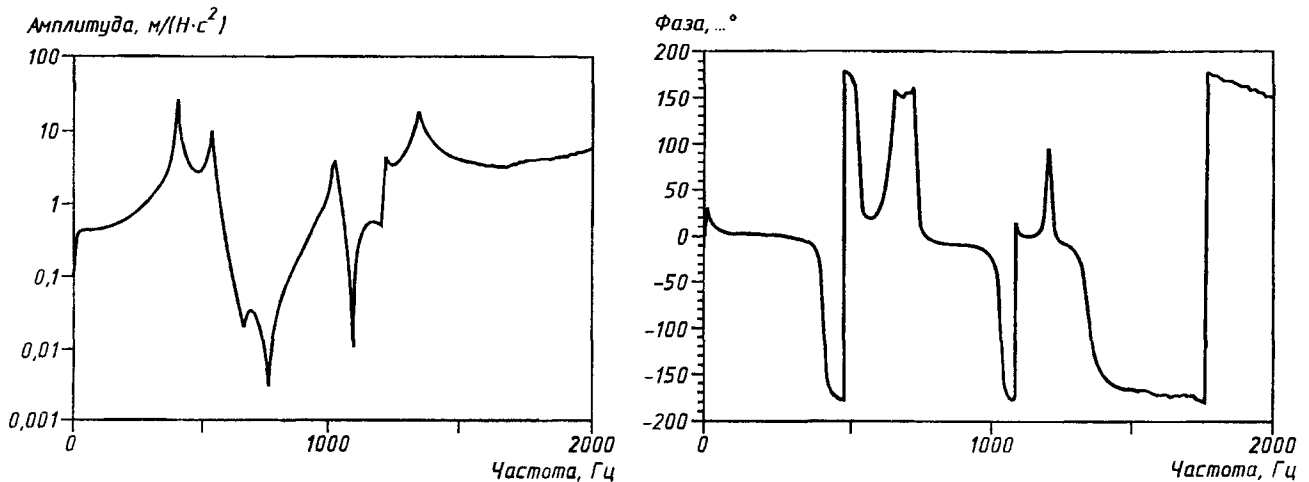
б) Ускоряемость, полученная после применения окна
