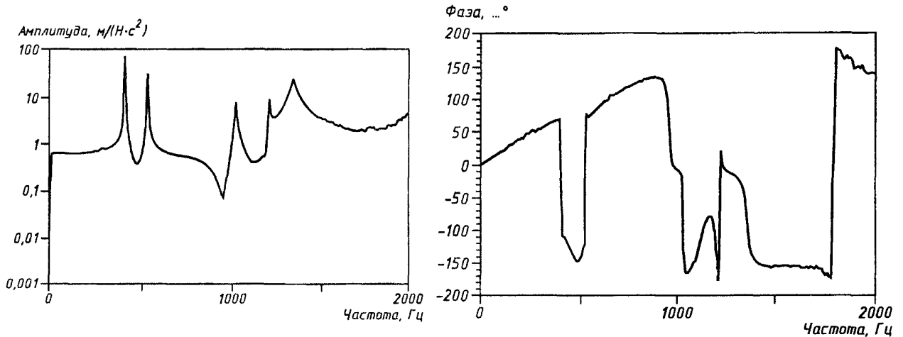
б) Ускоряемость (амплитуда и фаза) в отсутствие окна
