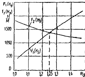
Рис. 7. Определение K_y методом Р. Р. Чугаева
