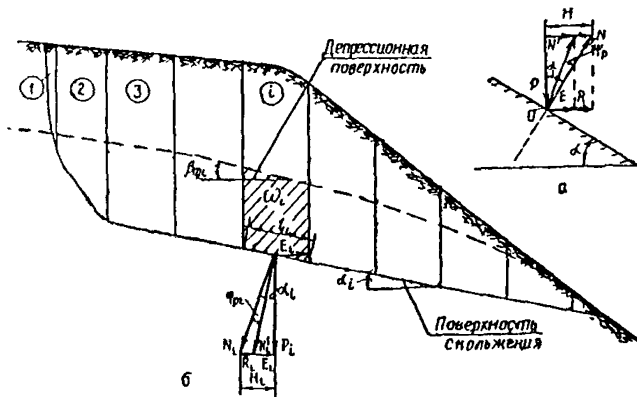
Рис. 8. Метод горизонтальных сил: а — основной принцип; б — использование для расчета устойчивости склона
