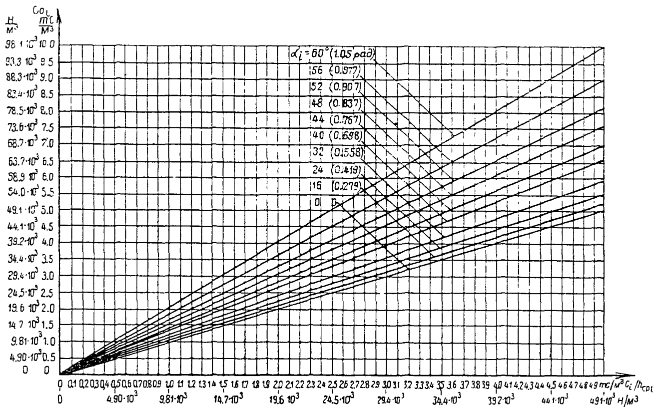
Рис. 14. Графики зависимости c_{oi} = \frac{c_i}{h_{cp} \cdot i \cos \alpha_i}
