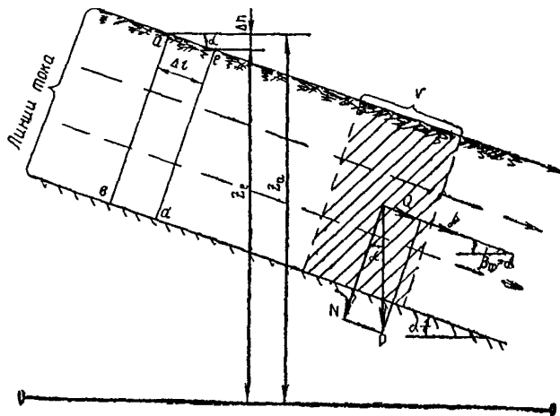
Рис. 1. Наклонный пласт водонасыщенного грунта
