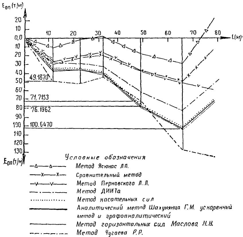
Рис. 24. Сравнение эпюр оползневого давления, рассчитанного различными методами
