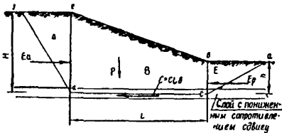
Рис. 17. Метод блока и призм (расчетная схема)
