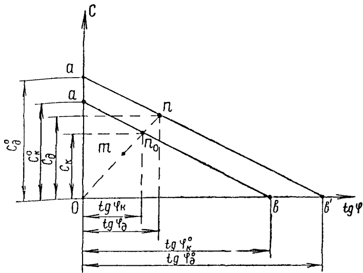
Рис 5 Кривые связи
