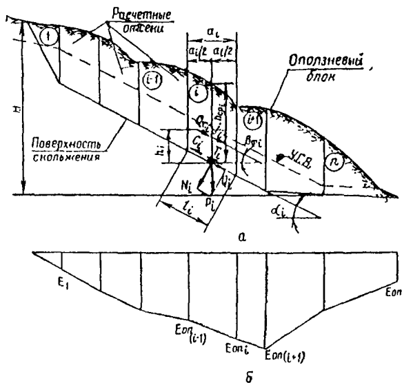
Рис. 12. Ускоренный способ расчета методом Г. М. Шахунянца: а — общая расчетная схема склона; б — эпюра оползневое давления
