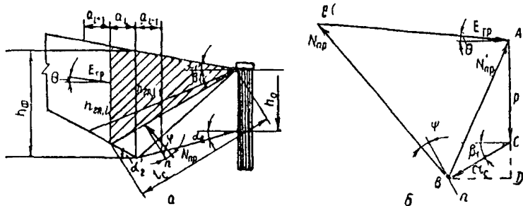
Рис. 22. Определение силы выпора: а — схема клина выпирания; б — силовой многоугольник
