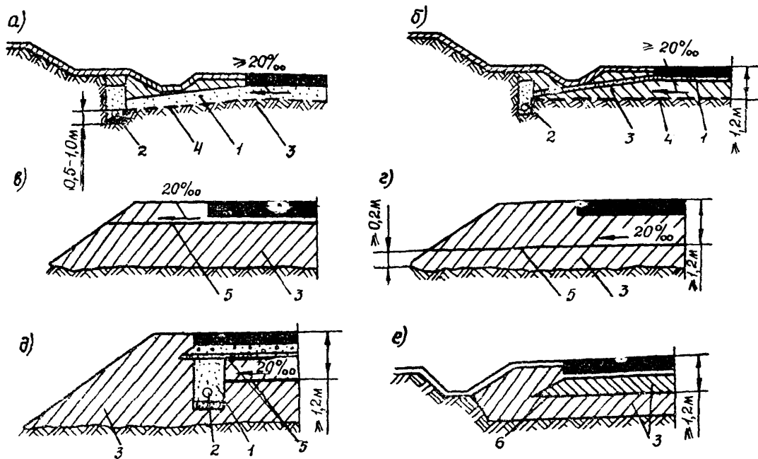
Рис.1. Конструкции земляного полотна с дренирующими, армирующими, капиллярно-прерывающими и гидроизолирующими прослойками: а-с совмещенной дренирующей и армирующей прослойкой; б-с капиллярнопрерывающей прослойкой; в,г,д,е-с гидроизолирующими прослойками; 1-песок; 2-трубчатый дренаж; 3-глинистый грунт; 4-материал типа "бидим"; 5-изол или полиэтиленовая пленка; 6-мастичная типа а колетанш
