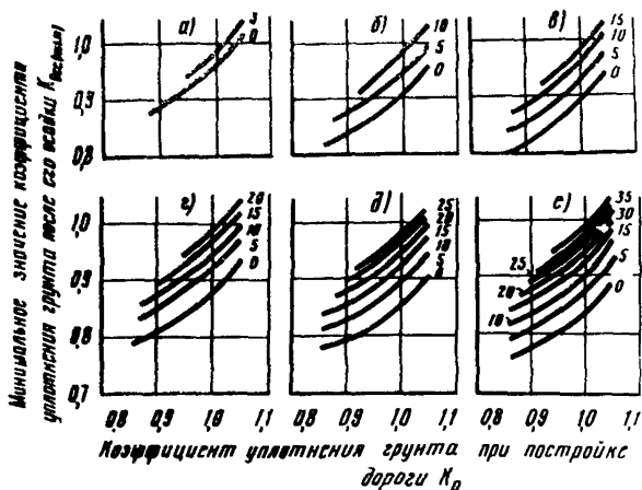
Рис.17. Графики для определения минимального коэффициента уплотнения грунта после осадки мелкого песка (а); пылеватого песка (б); пылеватой супеси (в); легкого суглинки (г); тяжелого суглинки (д); пылеватой глины (е). Цифры на кривых – давление на грунт, кПа
