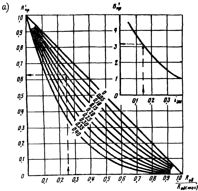
Рис.10. Номограммы для определения параметров A'_{sp} , промерзания грунта. Цифры на кривых - количество
