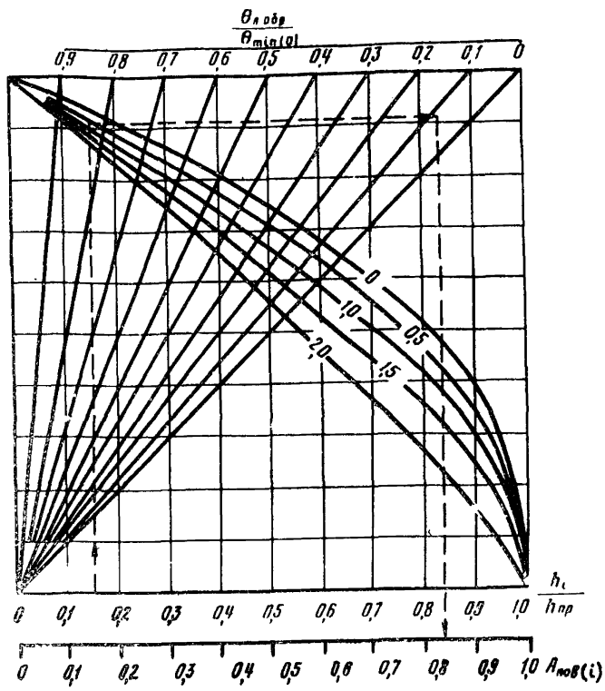
Рис.14. Номограмма для определения параметра A_{nob(i)} , входящего в расчет продолжительности периода повышения температуры грунта. Цифры на кривых - температура льдообразования
