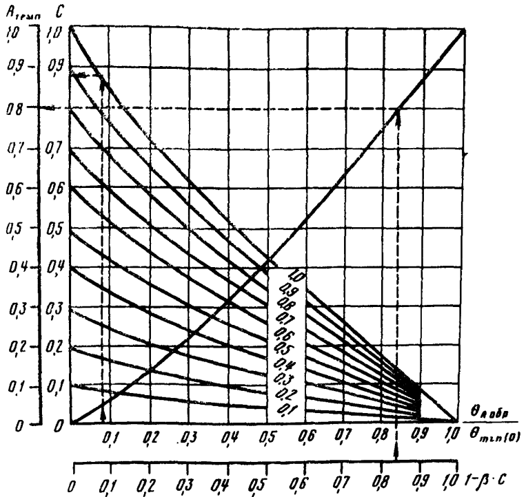
Рис.9. Номограмма для определения параметров C и A_{TEMP} , входящих в расчет глубины промерзания и температуры грунта. Цифры на кривых - отношение h_i/h_{пр} .
