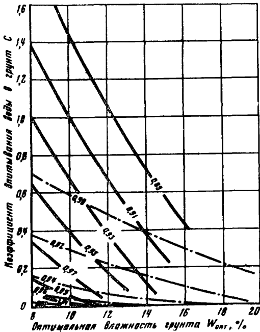
Рис.1. Номограмма для определения коэффициента впитывания воды в грунт земляного полотна C : — — — — — су-песи; - - - - - суглинки и глины. Цифры на кривых - коэффициенты уплотнения грунта
