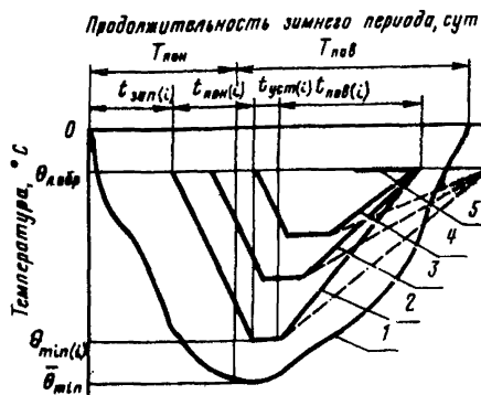
Рис.7. Расчетная схема температурного поля земляного полотна в зимний период: 1 - температура воздуха; 2 - ход температуры грунта на глубине h_i , м, от низа (каменной части) дорожной одежды; 3 - то же, на глубине h_{i+1} , т.е. ниже h_i ; 4 - то же, на глубине h_{i+2} , т.е. ниже h_{i+1} ; 5 - то же, на глубине промерзания за зиму, м (расстояние от низа каменной части дорожной одежды до глубины h_{пр} с температурой, равной температуре льдообразования).
