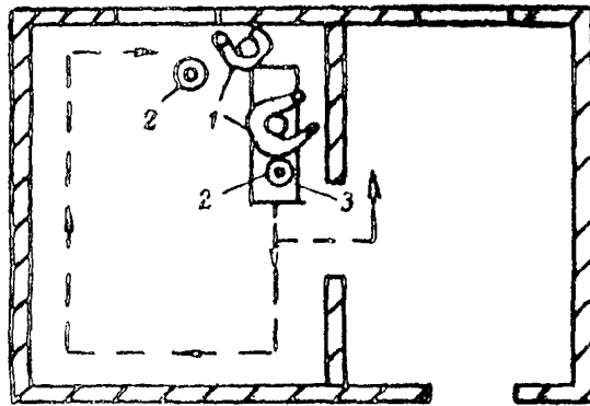
Шпатлевание поверхностей: 1 - маляры; 2 - емкость со шпатлевкой, 3 - столик- подмости
