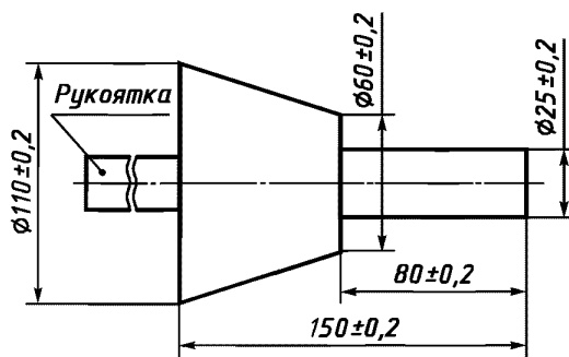
Рисунок 101 — Испытательный калибр
