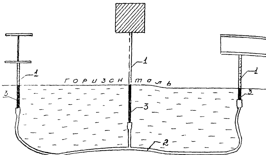
Рис.1. Схема гидравлического нивелирования:
