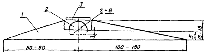
Рис.9. Устройство для определения давления колес крана:
