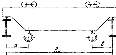
Рис.8. Схема расположения тележки
