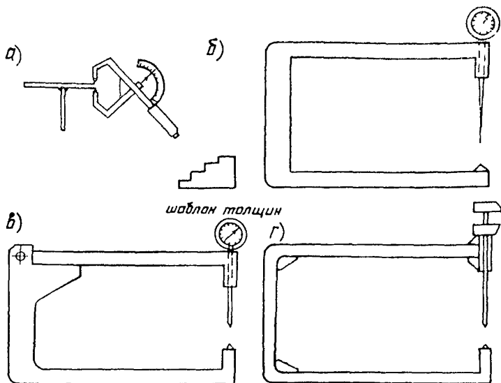
Рис.4. Инструменты для замеров толщины элементов:
