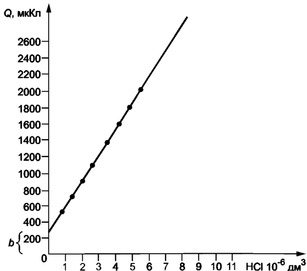
Рисунок 1 — Градуировочный график микрокулонометра
