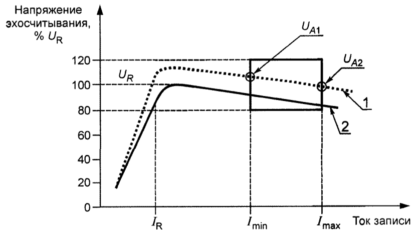
1 — кривая насыщения карты-образца; 2 — скорректированная кривая насыщения эталонной карты (приведена к первичному эталону)
