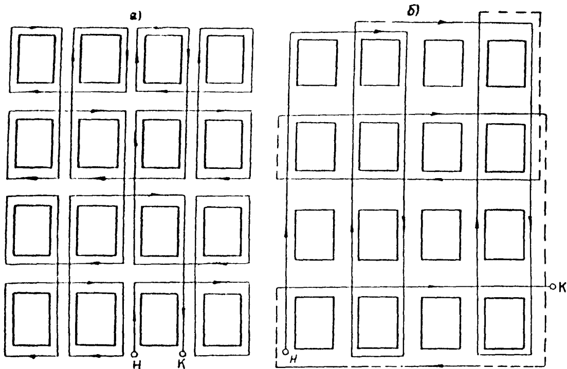
Рис. 2. Пример маршрута сбора ТБО с остановками для загрузки отходов: а - с одной стороны улицы (для улиц с двухсторонним движением); б - с двух сторон улиц (внутриквартальные провады); - - - - повторные проезды
