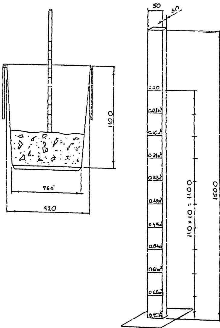
Схема рейки для определения объема твердых бытовых отходов в контейнере
