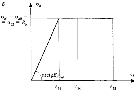
Рисунок 5.1 — Диаграммы состояния сжатого бетона
