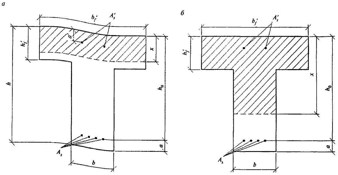
а — в полке; б — в ребре Рисунок 6.4 — Положение границы сжатой зоны в сечении изгибаемого железобетонного элемента
