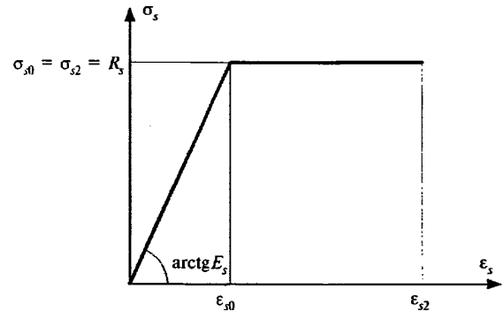
Рисунок 5.2 — Диаграмма состояния растянутой арматуры
