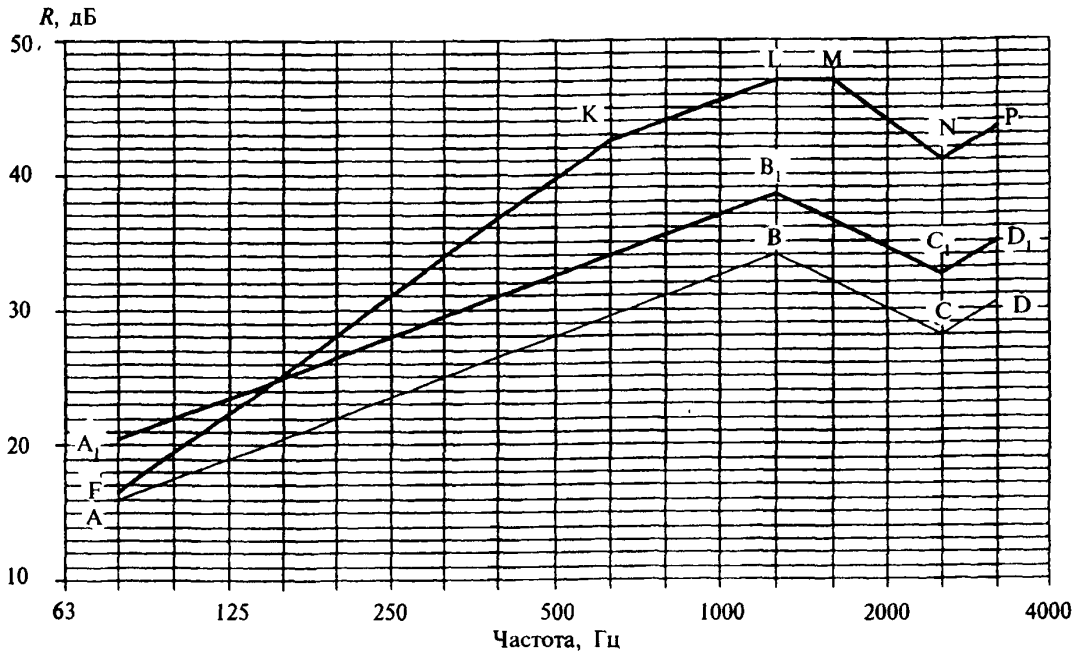
Рисунок 8 — Расчетная частотная характеристика к примеру 9
