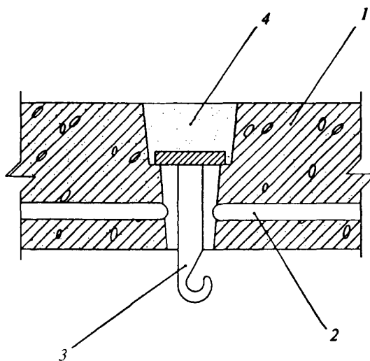
1 — панель перекрытия; 2 — электроканал; 3 — крюк, приваренный к круглой стальной пластине; 4 — раствор (заделка нижней части отверстия условно не показана)
