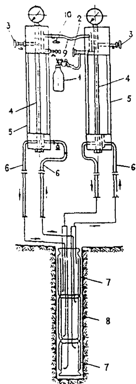
Рис.1. Схема прессиометра ПС-1 конструкции Фундаментпроект
