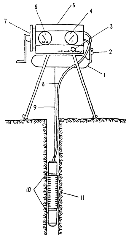
Рис.2. Схема прессиометра ИЦ-21 конструк- ции СКБ - ЗСЕГИНГЕО
