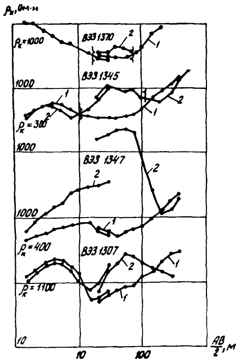
Рис. 3. Кривые крестовых зондирований на сквозных таликах в условиях бокового влияния мерзлых пород: 1 — линии разностей АВ вдоль талика; 2 — то же вкрест талика; --- — положение контакта мерзлых и талых пород
