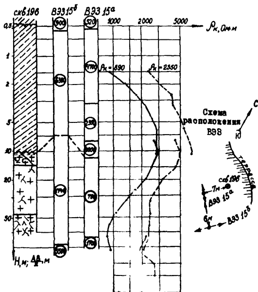
Рис. 12. Кривые ВЗВ, полученные у скважины № 196: - суглинки и глины мерзлые, в верхней части с прослойками льда; - гранит; - гранодиорит; - трещиноватость; - гранит сильно выветренный и заглинизированный; - верхняя (a) и нижняя (б) границы мерзлых пород
