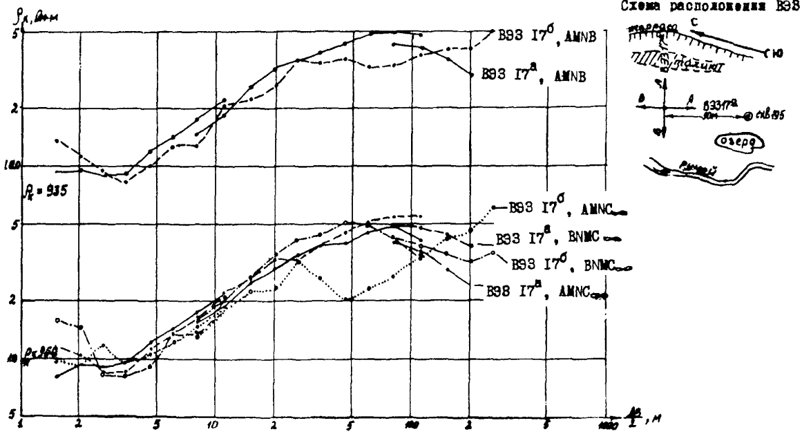
Рис. 13. Пример бокового влияния галых пород на результаты симметричного (AMNB) и трехполюсного (AMNC) ВЗБ
