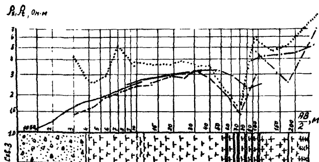
Рис. 6. Кривые \rho_k и \rho_t , полученные у скважины № 3 (по В.Я.Пригоде): [штрихованный квадрат] - моренные отложения; [квадрат с крестом] - биотитовые гнейсо-граниты; [квадрат с точками] - граниты; [квадрат с диагональными линиями] - гнейсифицированные гнейсы; [волнистая линия] - роговики; [квадрат с вертикальными линиями] - зоны повышенной трещиноватости и обводненности; [сплошная линия] - кривая \rho_k ; [пунктирная линия] - кривая \rho_t ; [дotted line] - кривая \rho_t , полученная в результате пересчета кривой \rho_k
