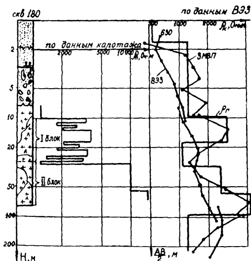
Рис. 9. Кривая ВЭЗ-13 б , полученная у скважины № 180;
