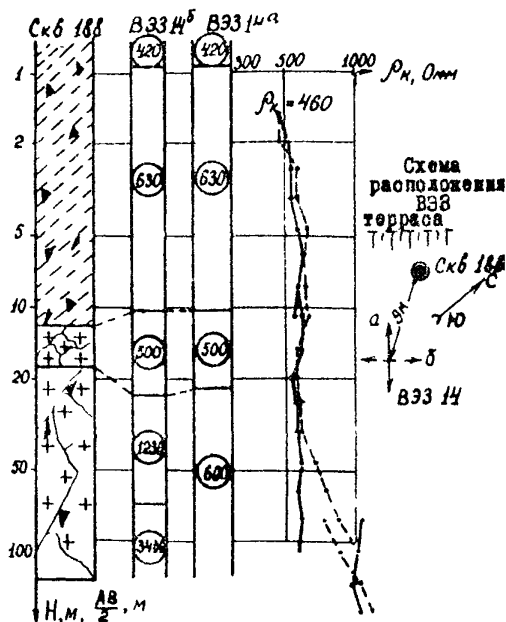
Рис. 11. Кривые крестового ВЭВ-14, полученные у скважины № 188:
