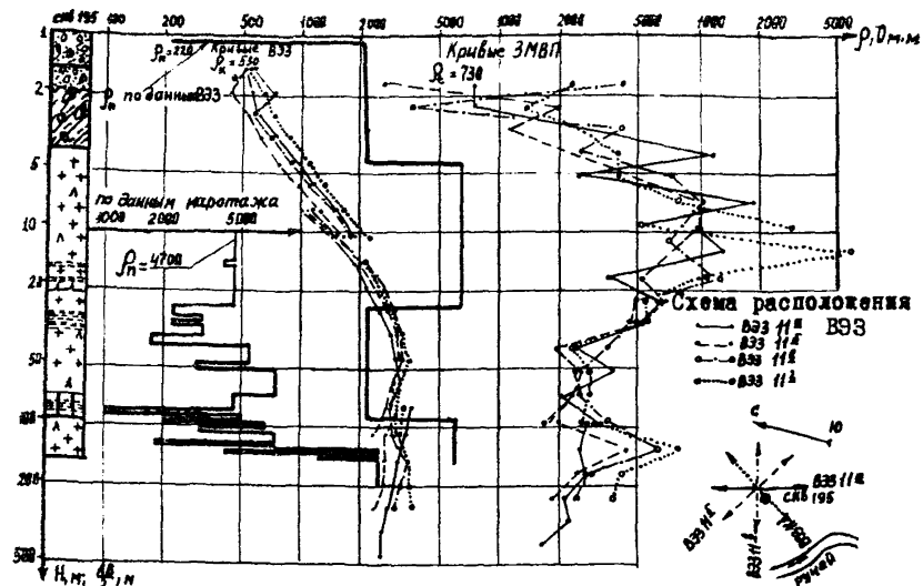
Рис. 8. Кривые \rho_k и \rho_t круговой В33-II, полученные у скважины № 195; - супесь с включением гравия и дресвы; - песок с галькой; - суглинок с древесной и воздушными коренными породами; - гнейсовидный гранодиорит; - наиболее трещиноватые породы по данным бурения; - зона максимального водопритока по данным каротажа; - верхняя (а) и нижняя (б) границы вечной мерзлоты
