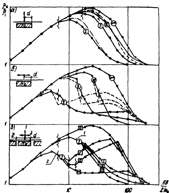
Рис. 1. Кривые ВЭЗ моделирования и графические кривые для случая зондирования над пластом мерзлых пород при боковом влиянии таликов (по С.А.Бойкову): а - вдоль границы; б - вкрест границы; в - вдоль (1) и вкрест (2) двух симметрично расположенных ограниченных таликов; — — — кривые моделирования; - - - - графические кривые; ②, ⑤, ⑩ и ⑳ - значения \frac{d}{P_2} ; [1], [2] - значения \frac{b-d}{P_2} ; — положение контакта мерзлых и талых пород; - мерзлые породы
