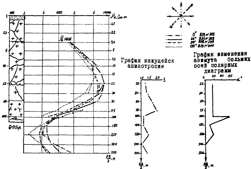
Рис. 16. Кривые круговых ВЗЗ и график кажущейся анизотропии, полученные у скважины № 262: [штриховка] - песок; [красный крест] - гранит; [зигзаг] - трещиноватость; [волнистая линия] - верхняя (а) и нижняя (б) границы вечной мерзлоты
