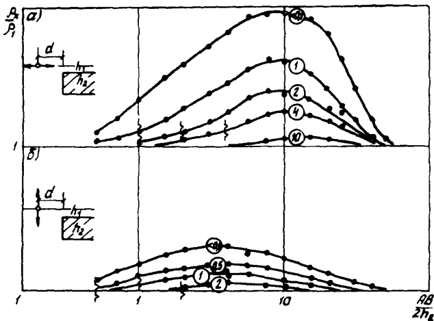
Рис. 2. Кривые ВЭЗ, полученные над моделью талика при боковом влиянии мерзлых пород (по С.А.Бойкову): ① — значения d/h_2 ; — положение контакта талых и мерзлых пород; ▨ — мерзлые породы; а — перпендикулярно контактам; б — параллельно контактам
