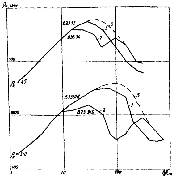
Рис. 5. Интерпретация кривых крестовых ВЭЗ по огибающей для случая бокового влияния тальных пород: 1 - экспериментальная кривая, полученная при разносах АВ вдоль границы раздела; 2 - то же при разносах АВ вкрат границе раздела; 3 - огибающая кривая
