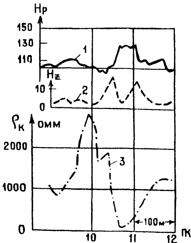
Рис. 3. Аномалии над закарстованной зоной известняков
