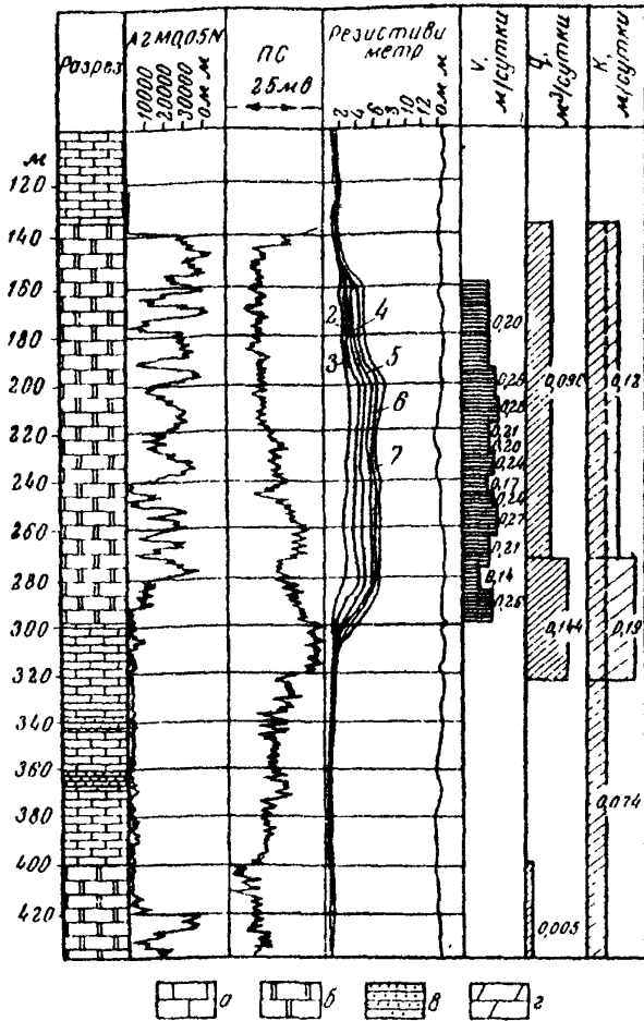
Рис. 7. Результаты исследований в скв. 466 Г (СУБР) 1 - кривая сопротивления воды до засоления; 2-7 - кривые после засоления (через каждые 60 мин); q - удельное водопоглощение; K - коэффициент фильтрации по данным налива; а - известняк; б - известняк кремнистый; в - сланец песчаный; г - доломит
