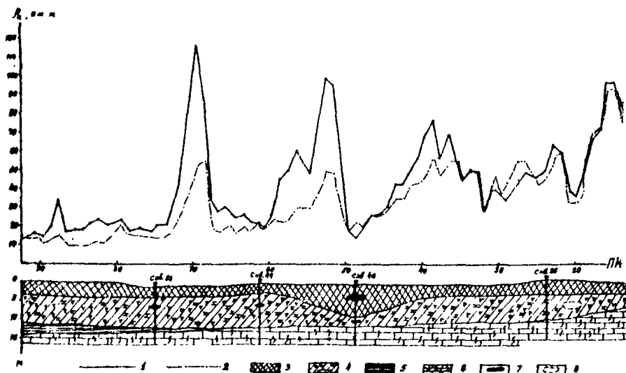
Рис. 9. Типичный график \rho_N и схематический геологический разрез ДСК г. Коломна
