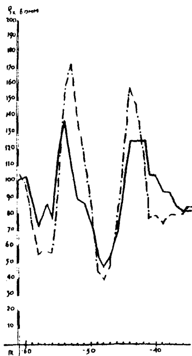
Рис. 5. Форма аномалии \rho_n в случае заполненной карстовой полости
