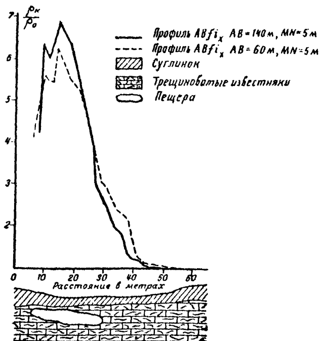
Рис. 4. Профиль сопротивлений по линии 1-1 (по А.М. Горелику)
