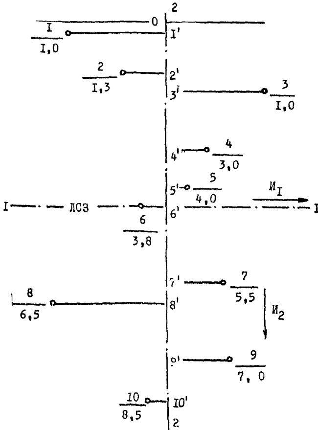
Рис. 2. Схема ключевой площадки с планом информативных точек (скважин): Числитель \Gamma - номер скважины, знаменатель - значения параметра \Pi ; 1' - 10' - проекции положения информативных точек на направление изменчивости \Pi_2(2-2) ; за начало отсчета(0) принято пересечение прямой 2-2 с границей поля
