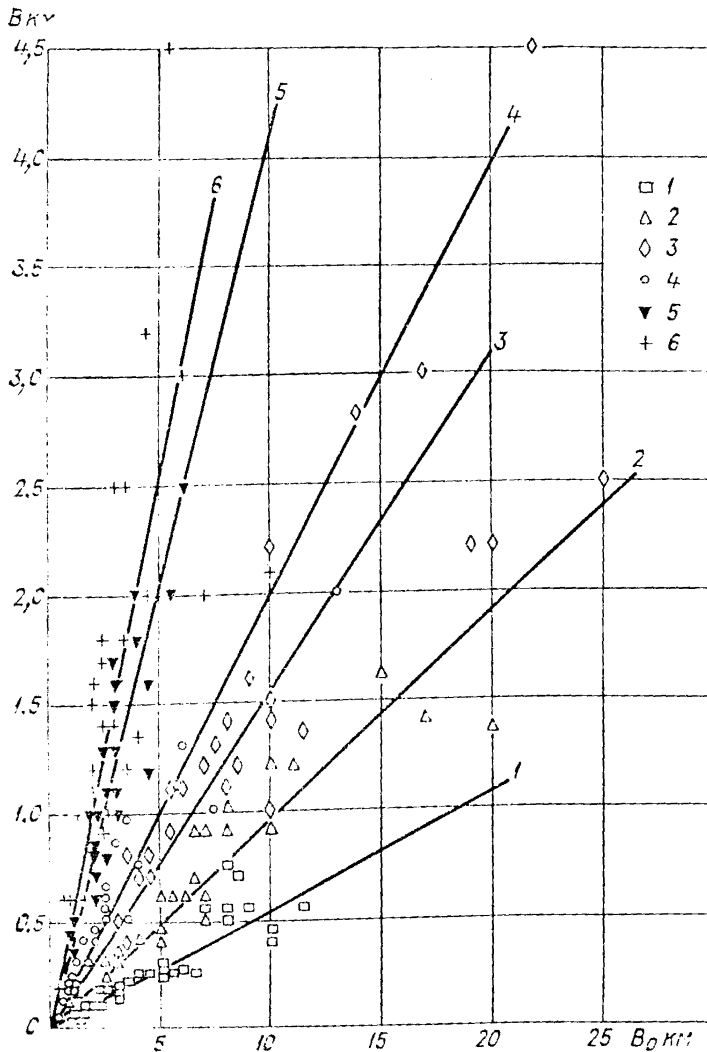
Рис. 9. Распределение типов руслового процесса в зависимости от ширины русла реки B и ширины долины B_0 .
