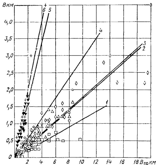
Рис. 10. Распределение типов руслового процесса в зависимости от ширины русла реки B и пояса руслоформирования B_{пр} .
