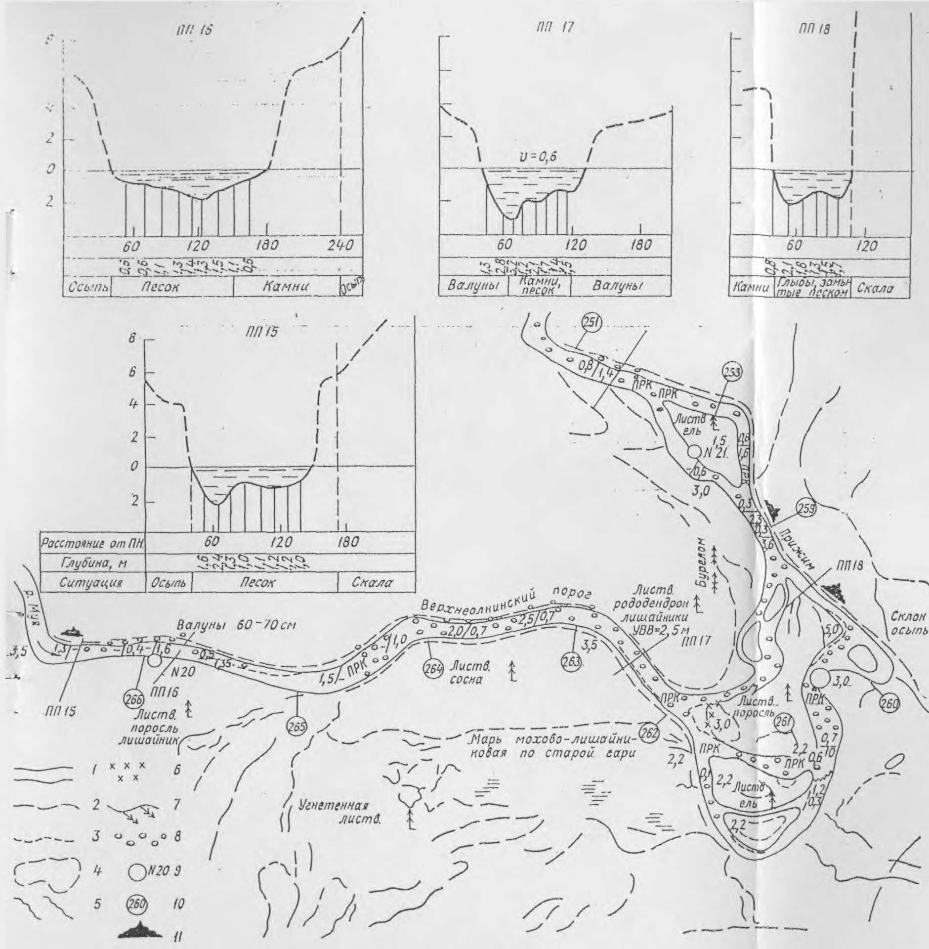
Рис. 7. Схема участка реки, полученная по материалам наземного обследования и аэрофотосъемки.
