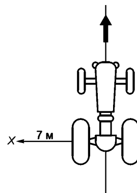
X — микрофон
