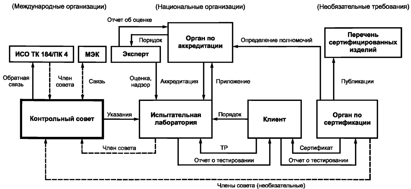
Рисунок D.1 — Инфраструктура аттестационного тестирования
