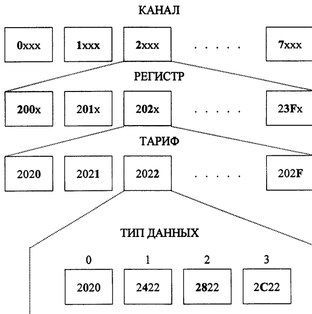
Рисунок В.2 — Диаграмма кодирования регистров
