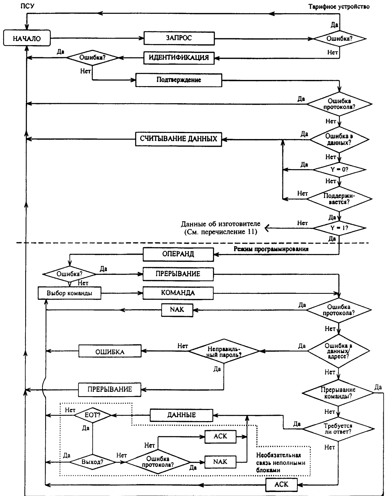
Блок-схема алгоритма для протокола прямого локального обмена данными, режим С
