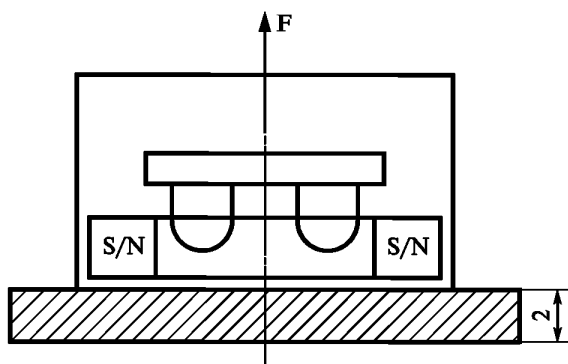
Рисунок 3а — Размещение магнита при определении силы сцепления
