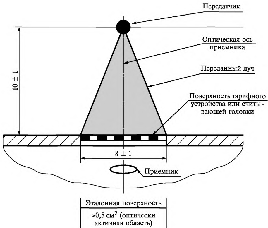
Рисунок 6 — Расположение приемника при испытаниях
