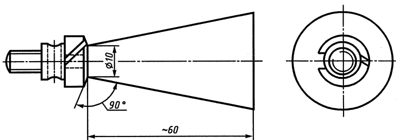
Рисунок 1 — Коническая оправка
