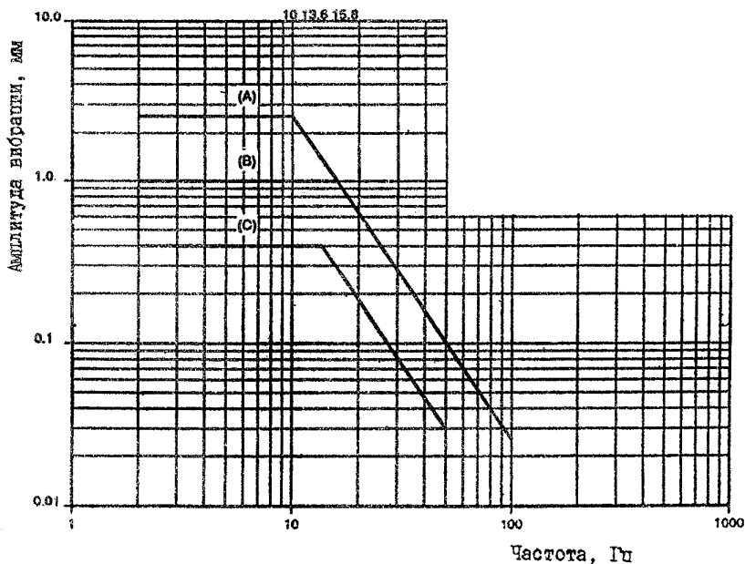
Рис. 19. Допустимые уровни вибрации оборудования СССР ИИМАРСАТ-С в зависимости от частоты
