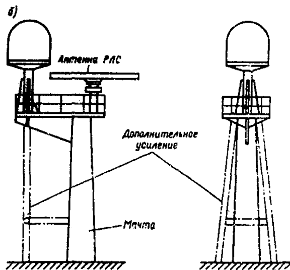
Рис. 2. Варианты установки антенного поста ССС:
