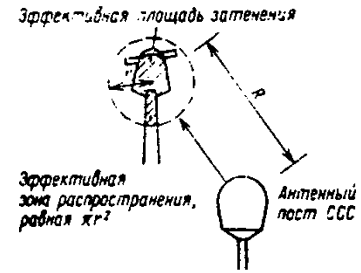
Рис. 11. Пример определения эффективной площади затенения для нецилиндрических препятствий: r — радиус эффективной зоны распространения; R — расстояние до препятствия
