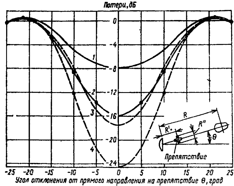
Рис. 8. Зависимость потерь усиления антенны от направления на препятствие в виде четырехугольной мачты и фальштрубы:
