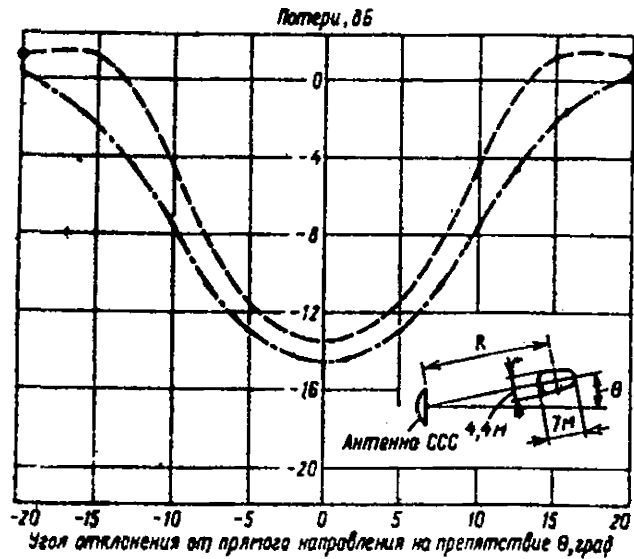
Рис. 6. Зависимость потери усиления антенны от направления на препятствие типа фальштрубы:
