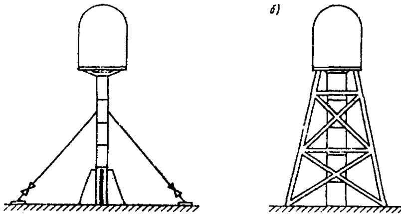
Рис. 1. Типы конструкций фундамента (опоры) для ССС: а — для установки антенны на высоте 2 м и менее над палубой; б — для установки антенны на высоте более 2 м над палубой
