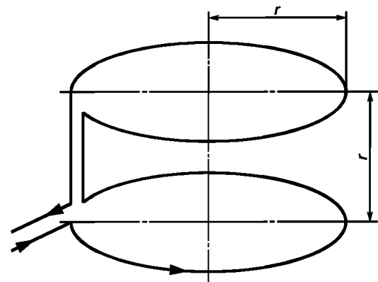
Рисунок Б.1 — Схема катушки Гельмгольца
