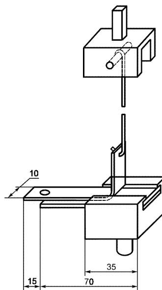
Рисунок 3 — Устройство для испытания образца
