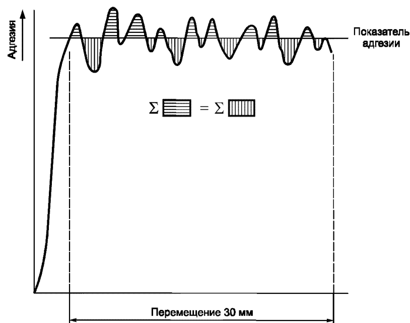
Рисунок 4 — Диаграмма «сила-перемещение»
