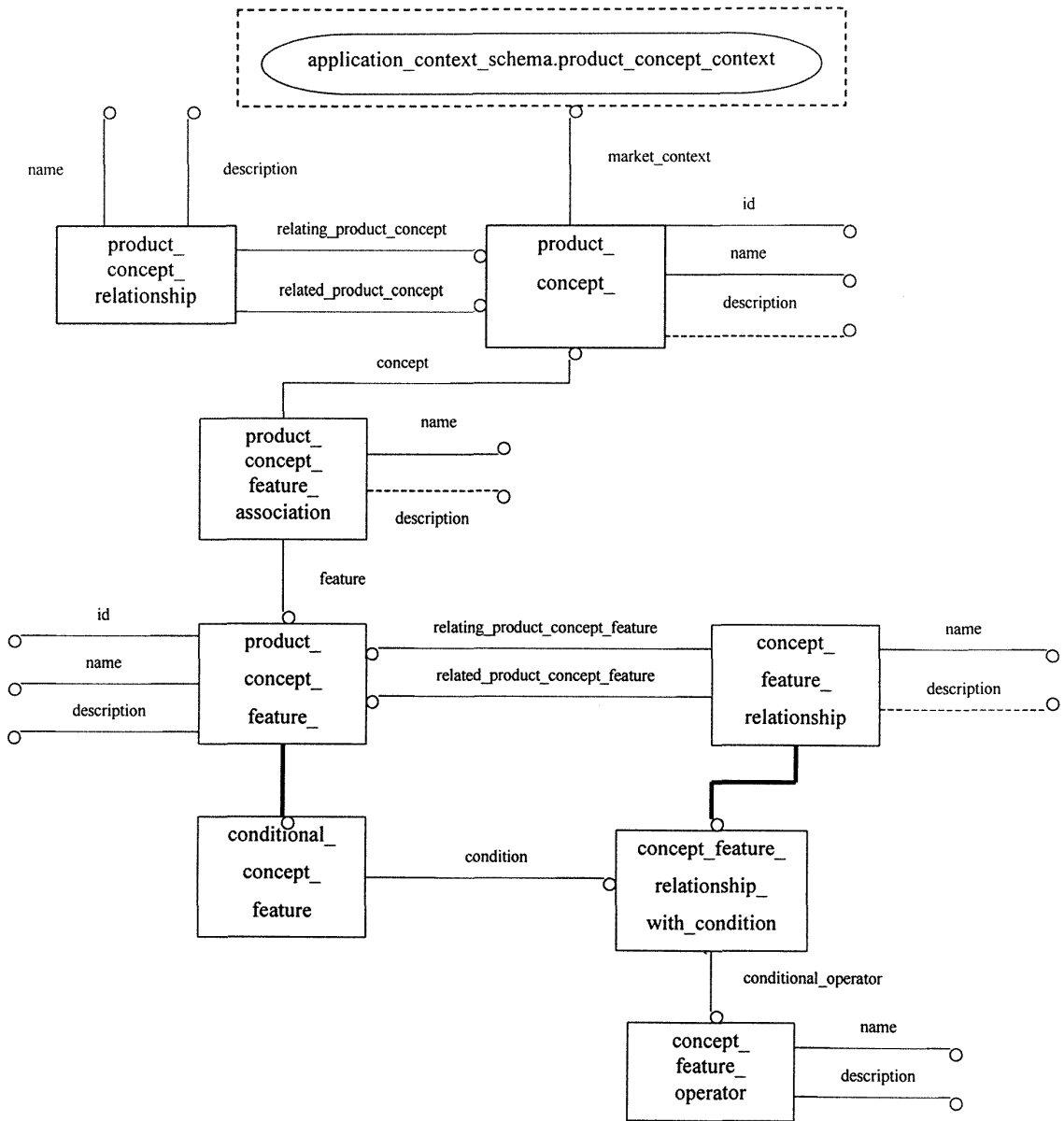
Рисунок D.2 — product_concept_schema
