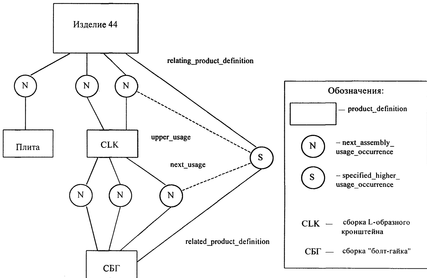
Рисунок Е.7 — Пример структуры данных списка частей с использованием объектов настоящего стандарта
