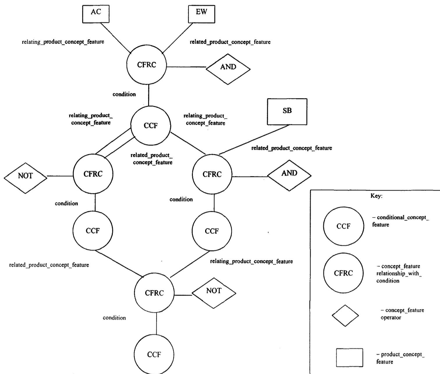
Рисунок Е.13 — Двоичные операторы для conditional_concept_feature
