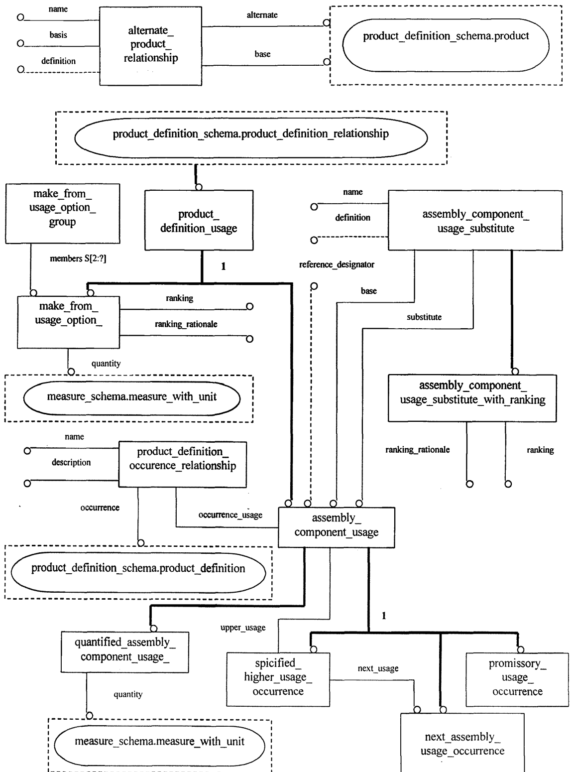
Рисунок D.1 — product_structure_schema
