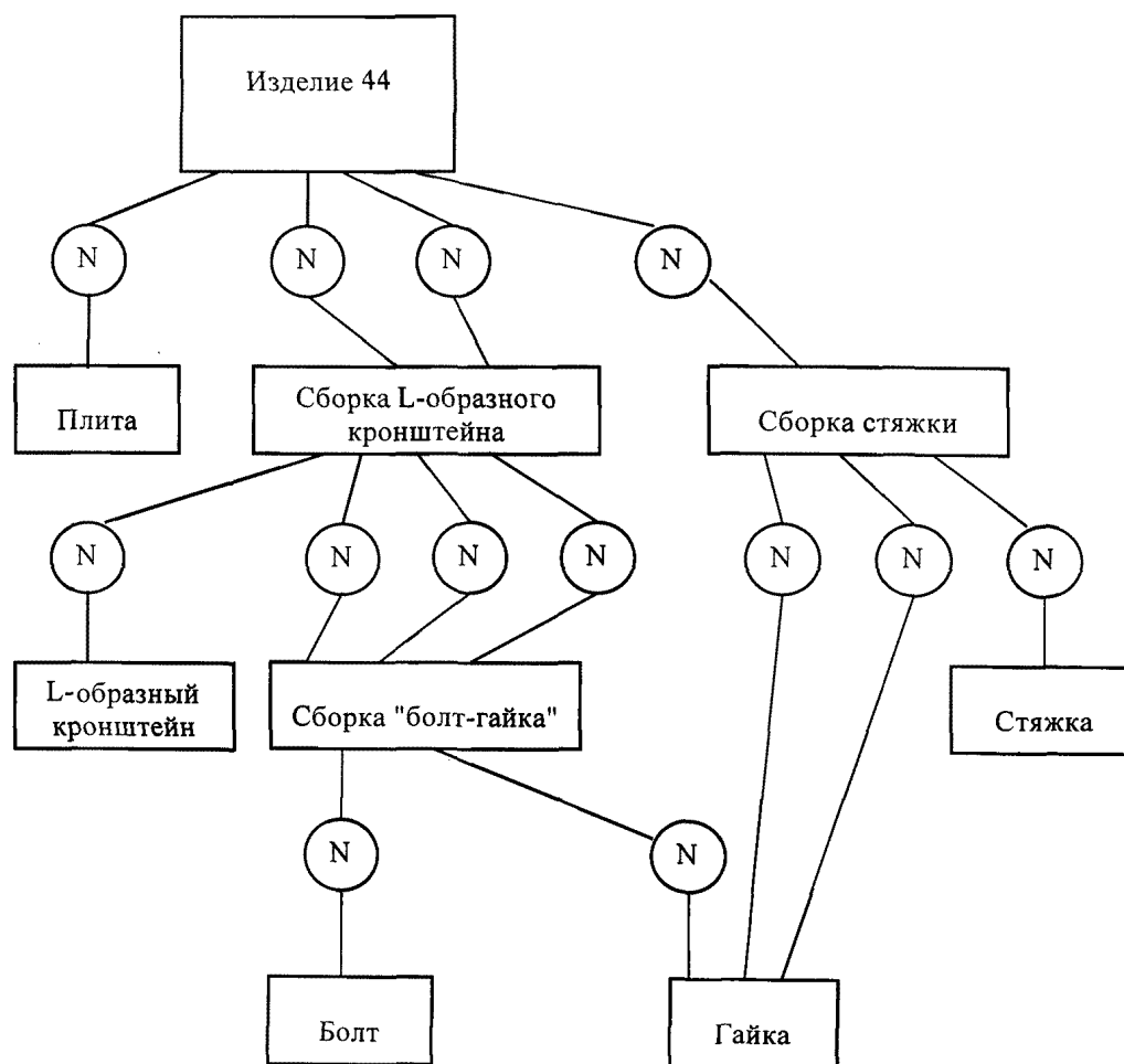
Рисунок Е.6 — Структура данных СП для изделия 44
