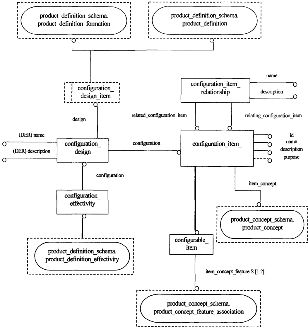
Рисунок D.3 — configuration_management_schema
