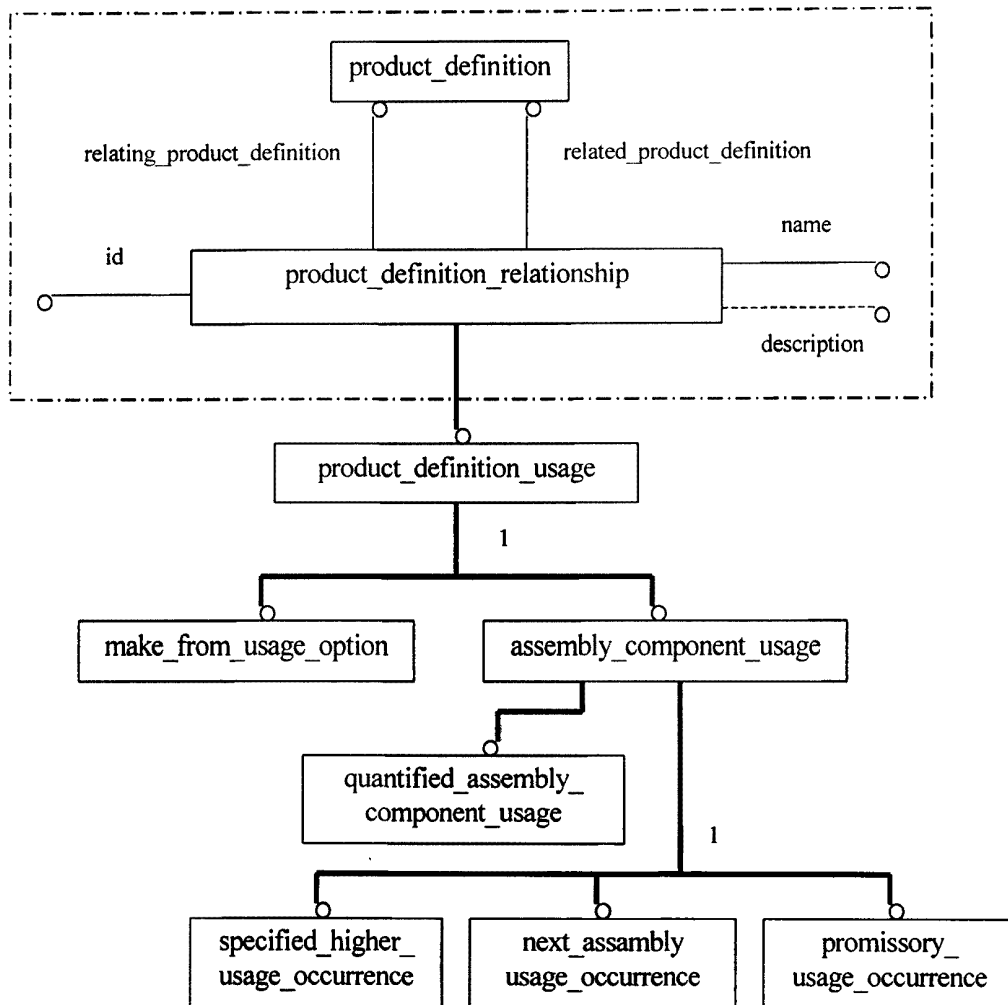
Рисунок 2 — Взаимосвязь объектов структуры изделия по ИСО 10303-41
