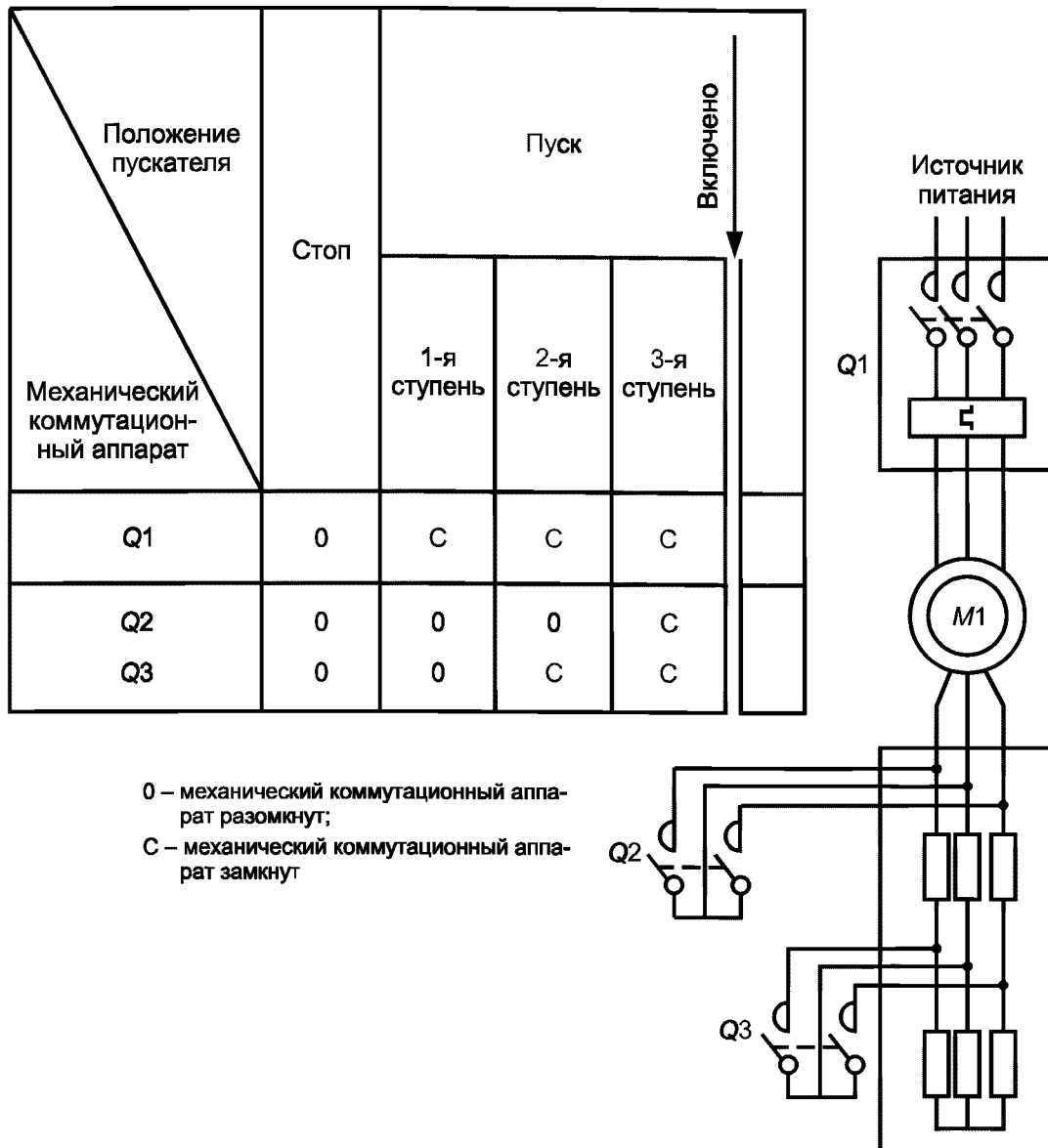
Рисунок 4 — Пример схемы трехфазного реостатного роторного пускателя с тремя пусковыми ступенями (см. 2.2.16) и одним направлением вращения (в случае, когда все механические коммутационные аппараты являются контакторами)
