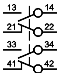
Четыре контактных элемента
