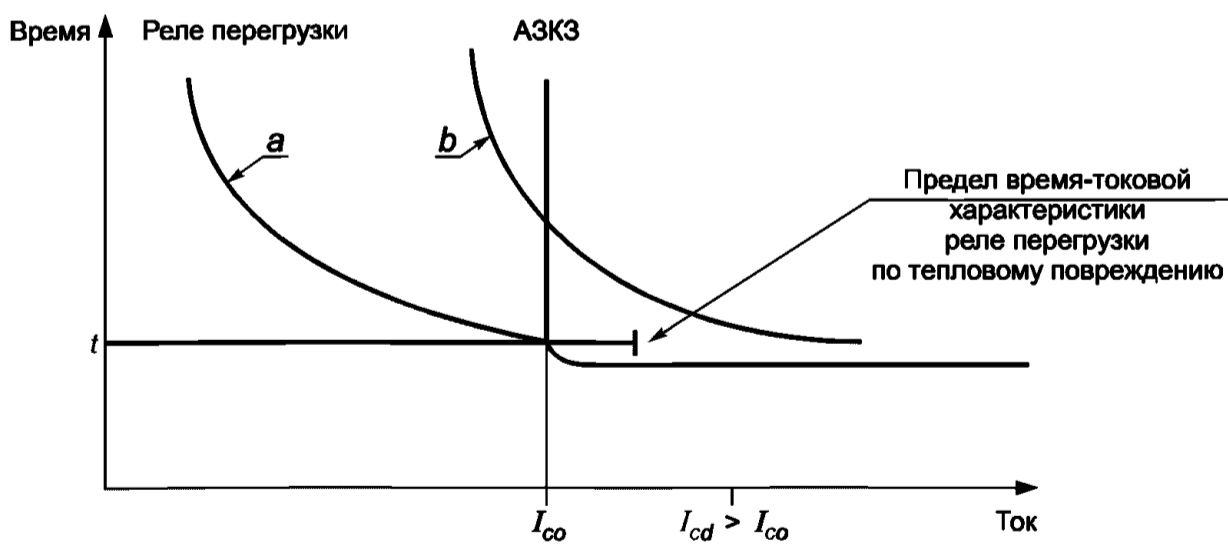
а) Координация с предохранителем
