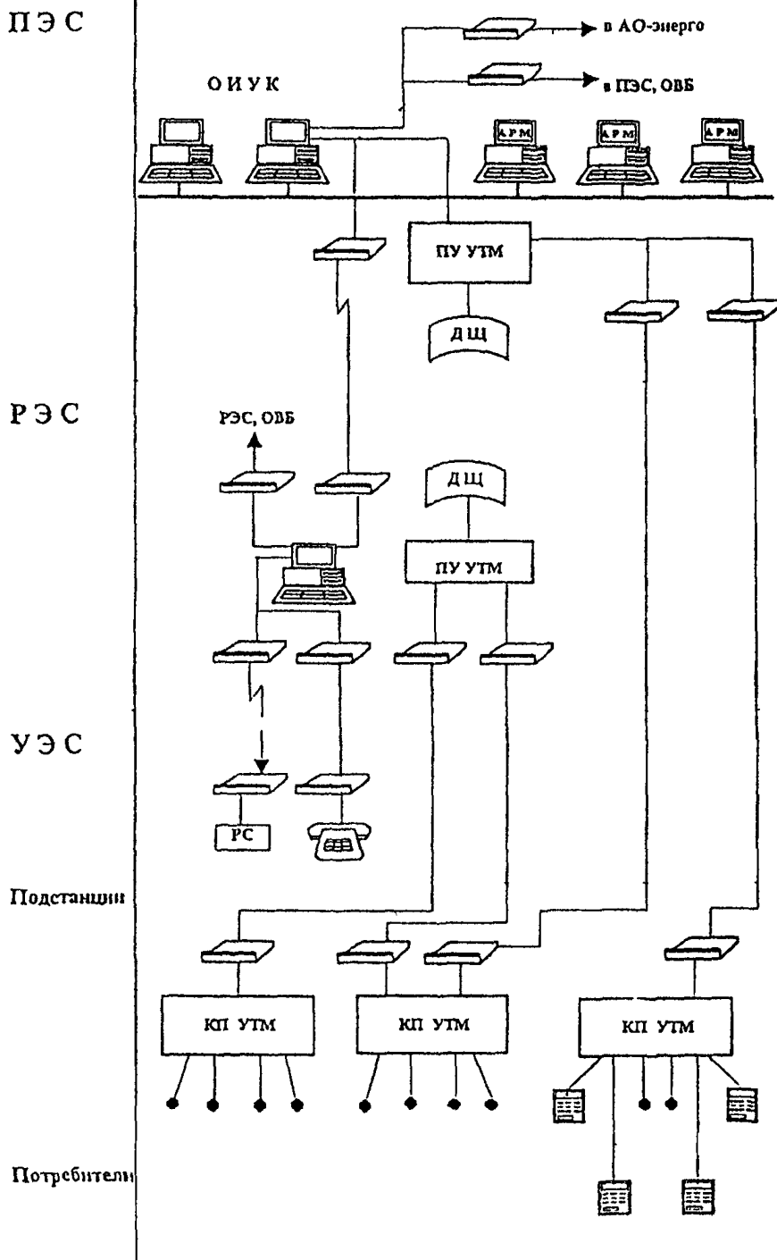
Рис 7. Архитектура первого этапа развития технических средств АСУ РЭС
