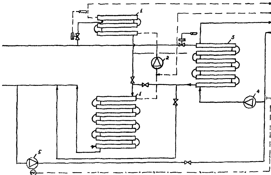
1 – подогреватель горячего водоснабжения № 12 ОСТ-34-588-68, I ступень – 7 секций, II ступень – 3 секции, 2 – циркуляционный насос К-90/20, 3 шт., 3 – подогреватель отопления № 14 ОСТ-34-588-68, 6 секций, 4 – отопительные насосы К-40/55А, 5 – подпиточный насос ВК 2х2В, 2 шт. Рисунок Р 1 – Принципиальная тепловая схема ЦТП
