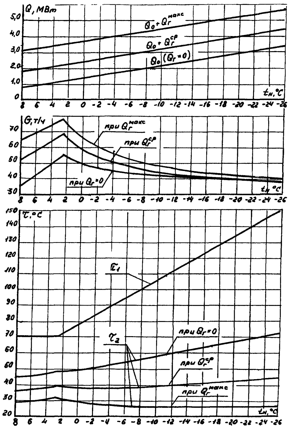
Рисунок Р 6 - Режимы работы ЦТП при проектных нагрузках Отопление Q_0 = 3,41 \text{ MBt} , средняя горячего водоснабжения Q_r^{\text{cp}} = 1,04 \text{ MBt}
