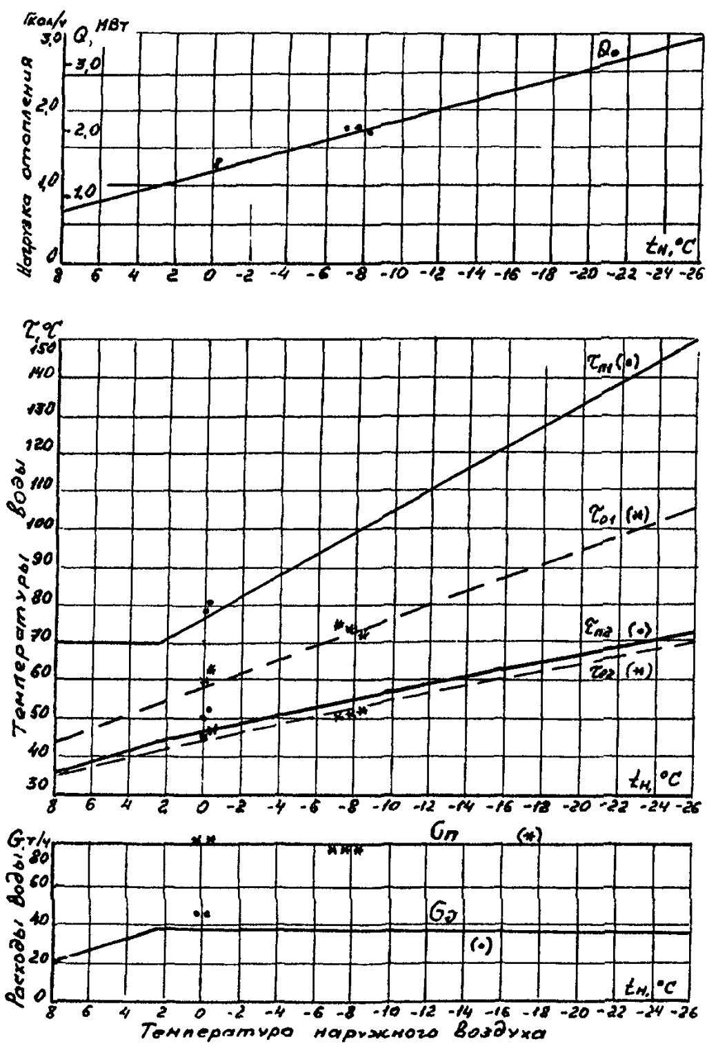
Рисунок Р 2 – Режимы работы системы отопления при проектной нагрузке Q'_0=3,41 \text{ MW}
