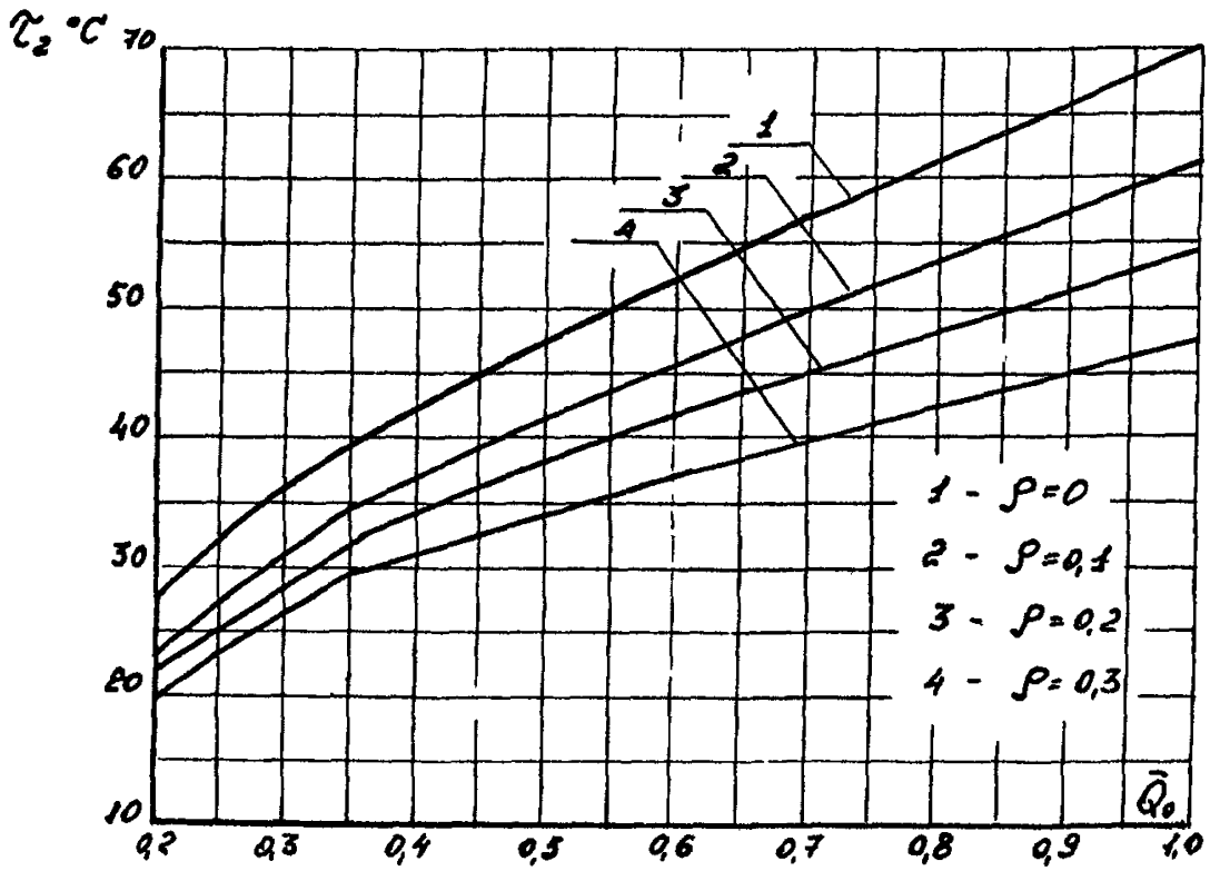
Рисунок 12 лист 4 Температурный график повышений рассчитанный на \mu = 0,3
