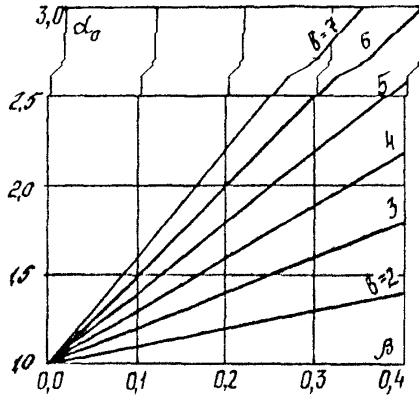
Рис.7. Зависимость поправочного коэффициента \alpha_0 от \beta и \theta
