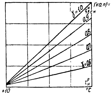
Рис.5. Зависимость нормы расхода тепла на вентиляцию от t_H и \delta
