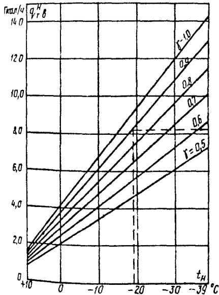
Рис. 18. Зависимость нормы расхода тепла на технологическую вентиляцию машинного отделения от t_H и \gamma
