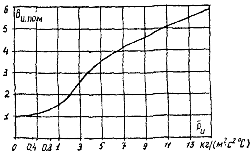
Рис.2. Зависимость коэффициента B_{u, пом} для помещения с двусторонним остеклением от относительного ветрового давления p_u [I]
