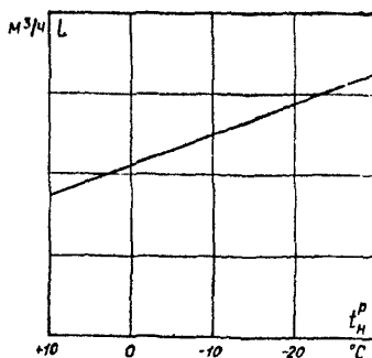
рис.3. Зависимость расчетного расхода воздуха на приточные установки с калориферами "на протос"
