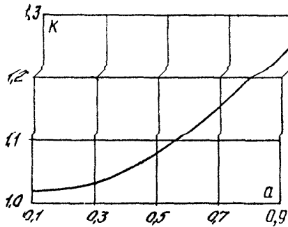
Рис.8. Зависимость коэффициента K от a
