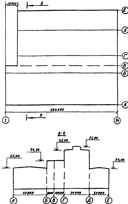
Рис.10. Главный корпус ТЭС в плане и разрезе
