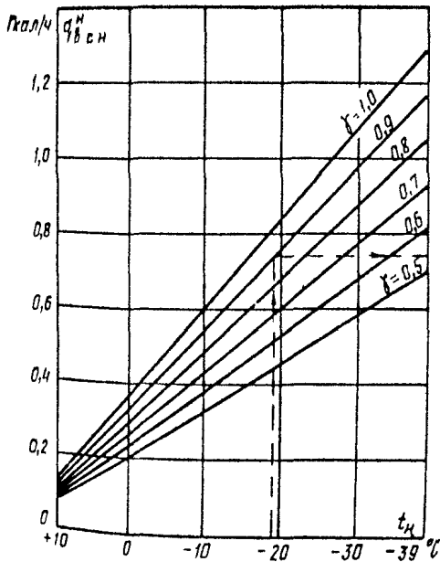
Рис.14. Зависимость нормы расхода тепла на вентиляцию котельного отделения от t_H и \gamma
