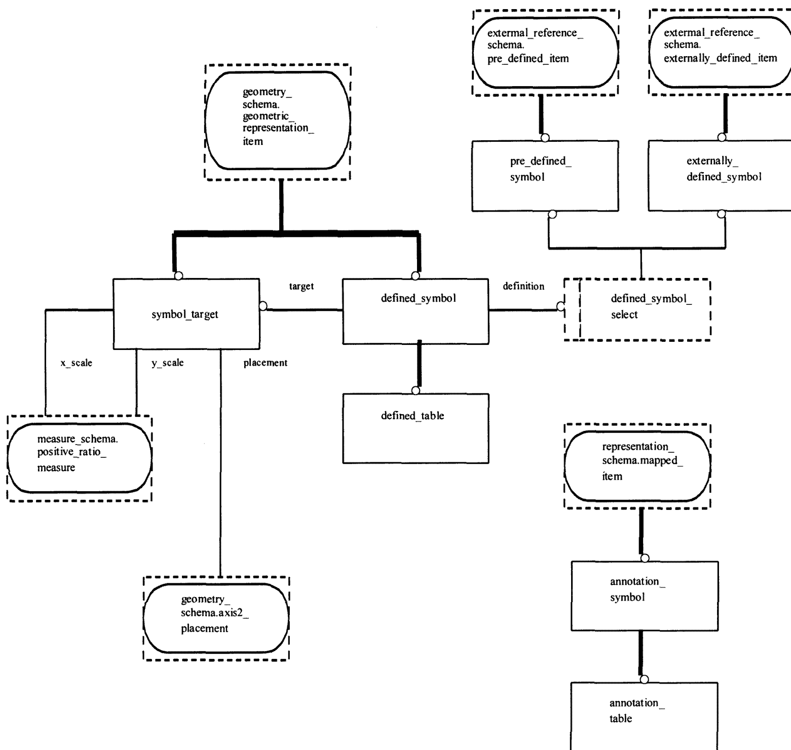
Рисунок Е.9 — EXPRESS-G диаграмма presentation_definition_schema 2 из 9
