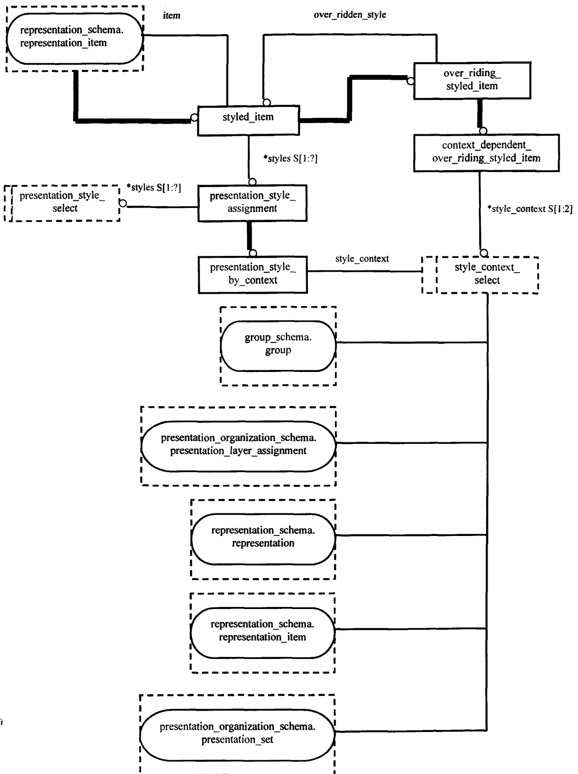
Рисунок Е.17 — EXPRESS-G диаграмма presentation_appearance_schema 1 из 21
