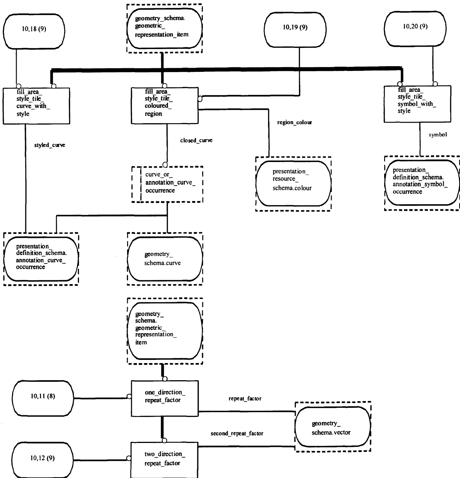
Рисунок Е.26 — EXPRESS-G диаграмма presentation_appearance_schema 10 из 21
