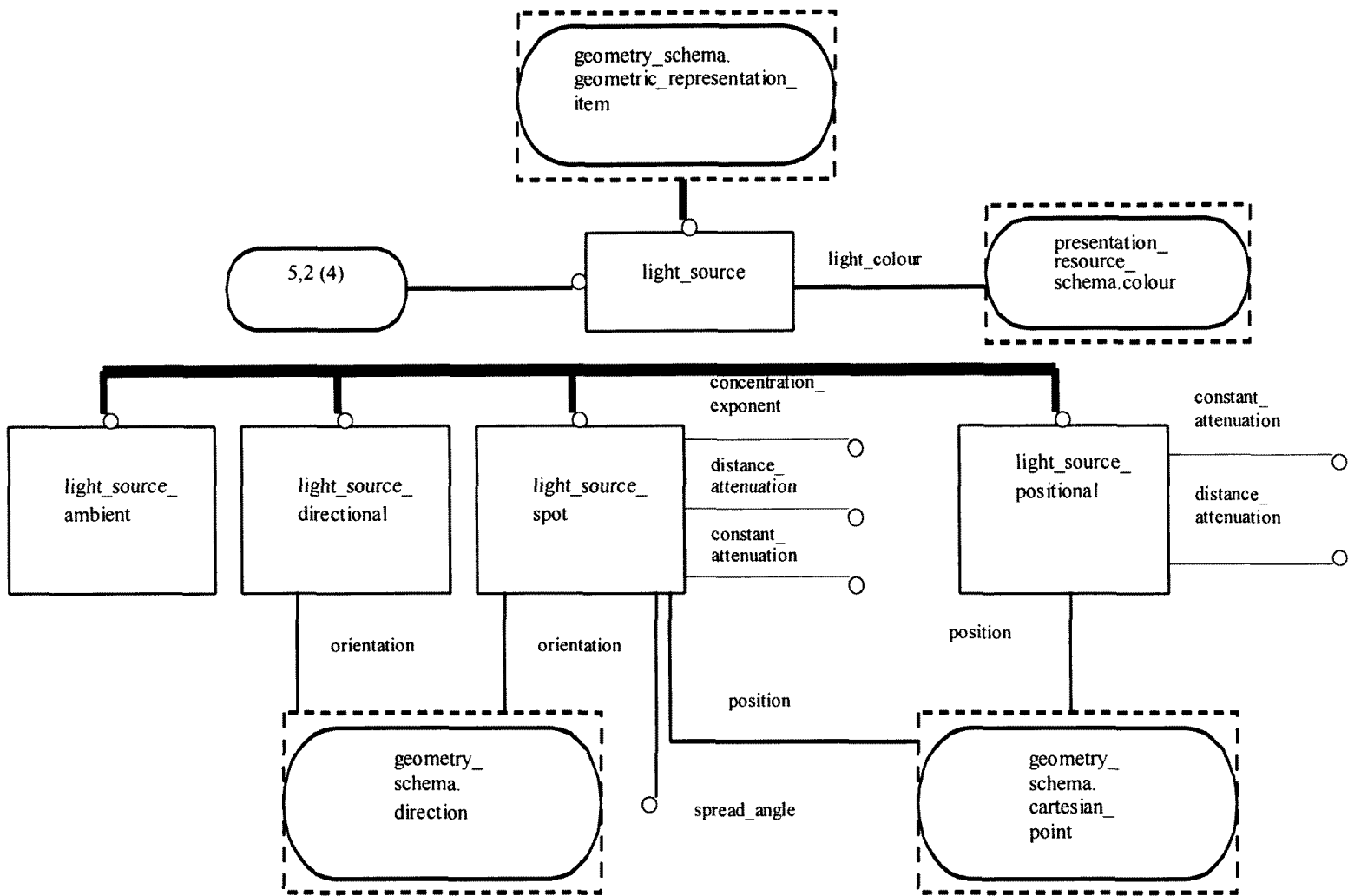
Рисунок E.5 — EXPRESS-G диаграмма presentation_organization_schema 5 из 7
