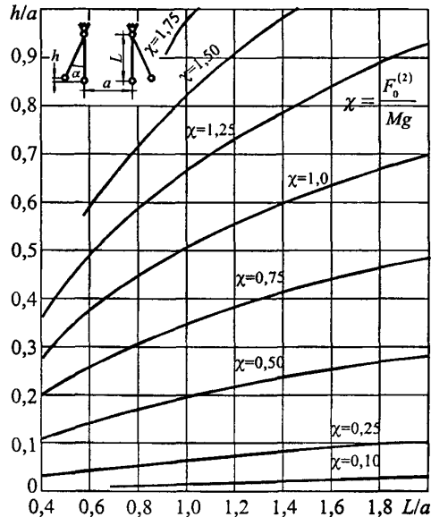
Рис. 7.12. Характеристики h/a при двухфазном КЗ
