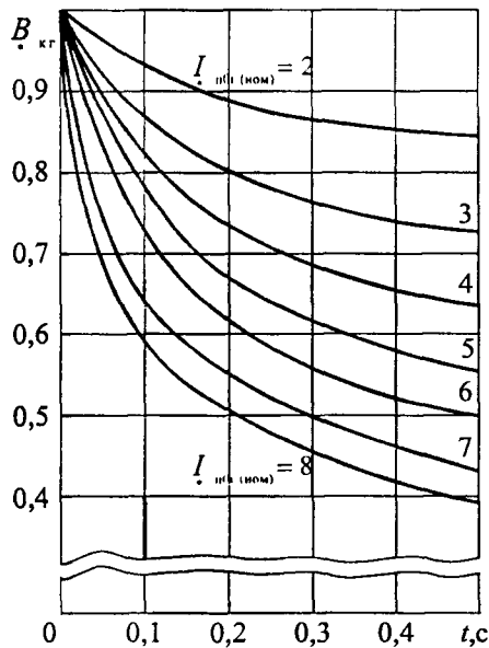
Рис. 8.2. Кривые для определения B_{кр} от синхронных генераторов с тиристорной системой возбуждения
