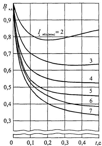
Рис. 8.4. Кривые для определения B_{кл} от синхронного электродвигателя
