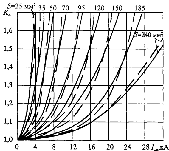
Рис. 5.23. Зависимость K_\phi = f(I_{но}, S_{но}) для кабелей с алюминиевыми жилами с учетом теплоотдачи и сопротивления дуги
