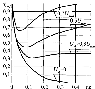
Рис. 5.16. Расчетные кривые для асинхронного электродвигателя
