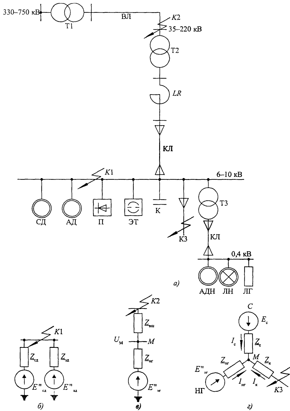
Рис. 5.14. Схема узла комплексной нагрузки и ее преобразование
