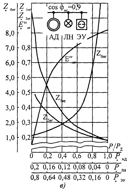
Рис. 6.6. Зависимость параметров комплексной нагрузки Z_{1нр} , Z_{2нр} , Z_{0нр} , E''_{нр} от ее состава
