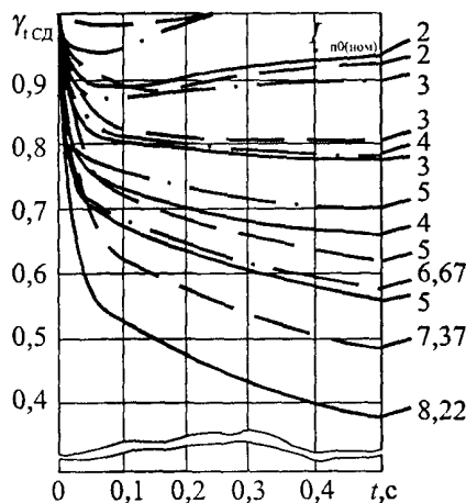
Рис. 5.10. Типовые кривые изменения тока КЗ от синхронных электродвигателей серии СДН (сплошные линии), серии СД с частотой вращения 1500 об/мин (штрихпунктирные линии) и серии СТД (пунктирные линии со звездочками)
