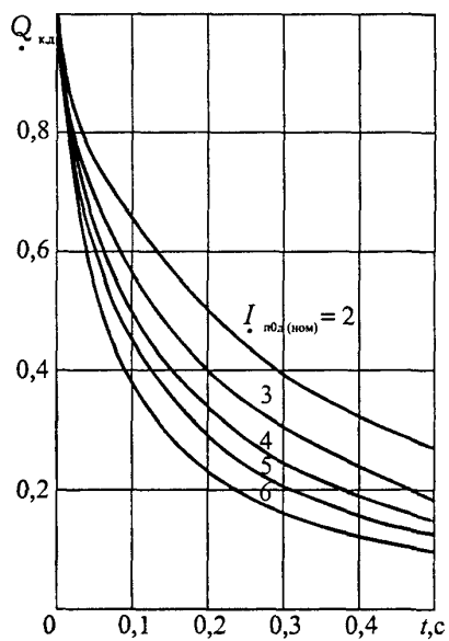
Рис. 8.7. Кривые для определения Q_{кл} от асинхронного электродвигателя
