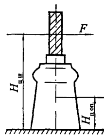
Рис. 7.8. К расчету приведенной массы опоры
