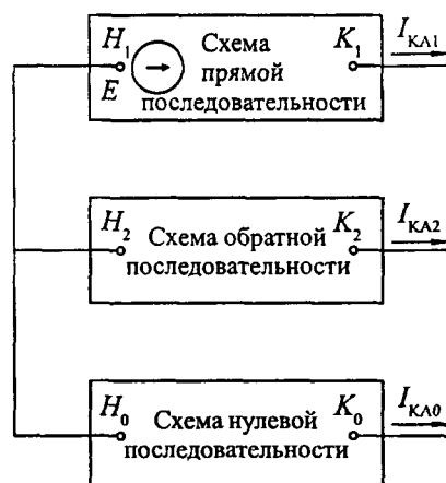
Рис. 3.4. Комплексная схема замещения для двухфазного КЗ на землю
