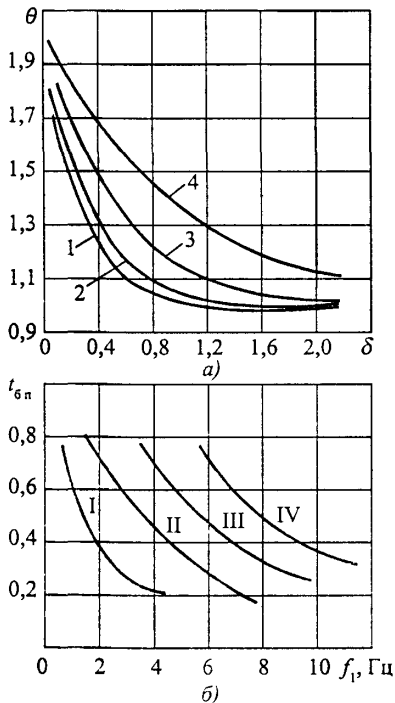
Рис. 7.9. К определению коэффициента превышения \theta в зависимости от \delta, t_{\text{он}}, f_1
