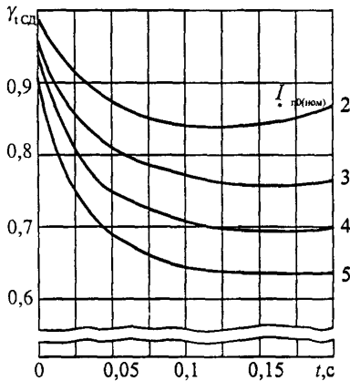
Рис. 5.8. Типовые кривые для синхронного электродвигателя
