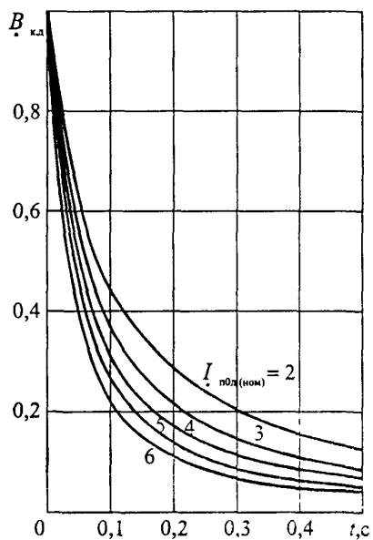
Рис. 8.6. Кривые для определения B_{кл} от асинхронного электродвигателя
