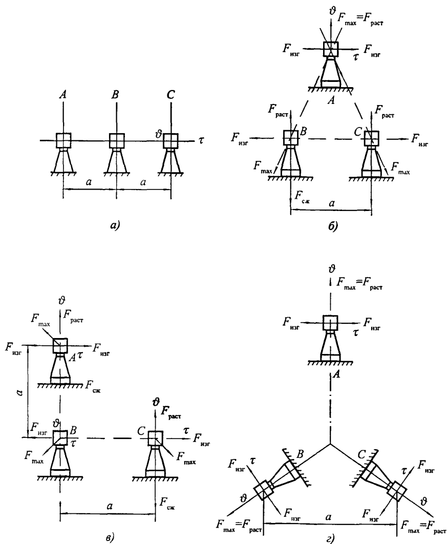
Рис. 7.2. Схемы взаимного расположения шин
