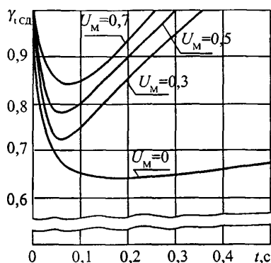
Рис. 5.15. Расчетные кривые для синхронного электродвигателя
