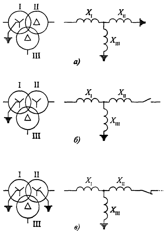
Рис. 3.2. Схемы замещения нулевой последовательности трехобмоточных трансформаторов
