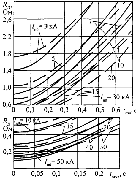
Рис. 5.20. Зависимость R_d = f(t_{откл}, I_{n0}) при КЗ на воздушных линиях 110 кВ (сплошные кривые) и 220 кВ (пунктирные кривые)
