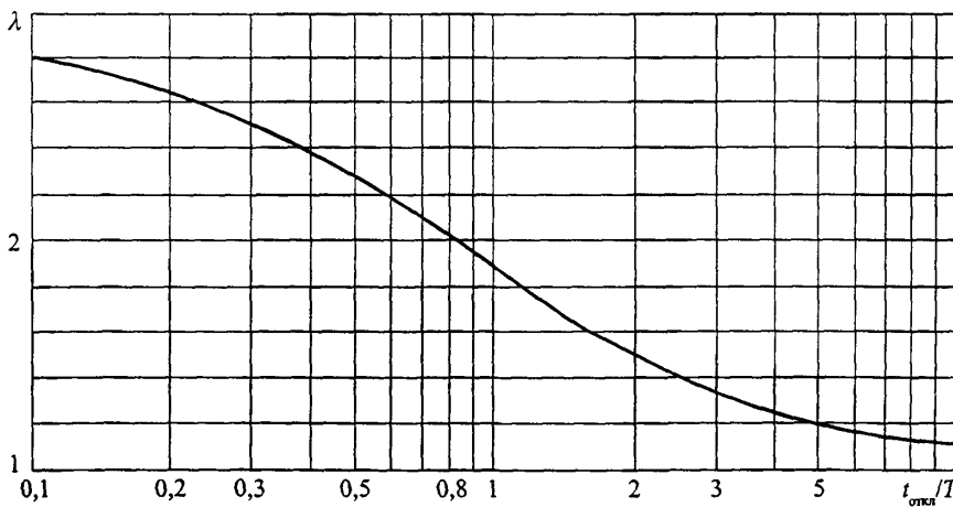
Рис. 7.10. Зависимость коэффициента приведения электродинамической нагрузки \lambda от t_{\text{откл}} / T_z .
