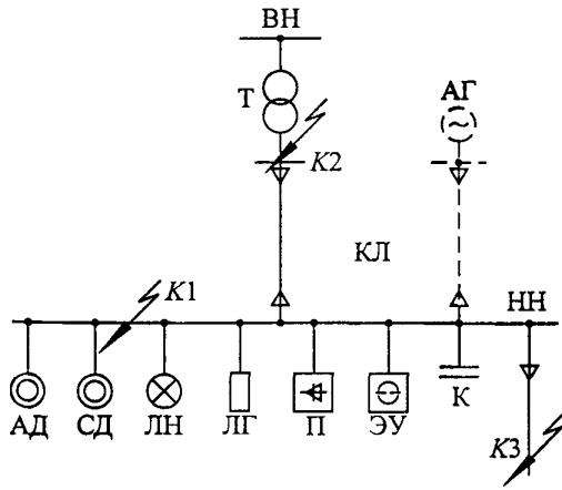
Рис. 6.7. Типовая расчетная схема узла комплексной нагрузки
