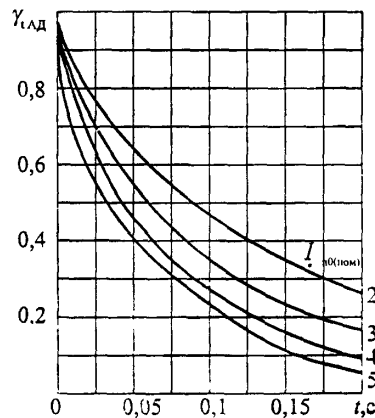
Рис. 5.9. Типовые кривые для асинхронного электродвигателя
