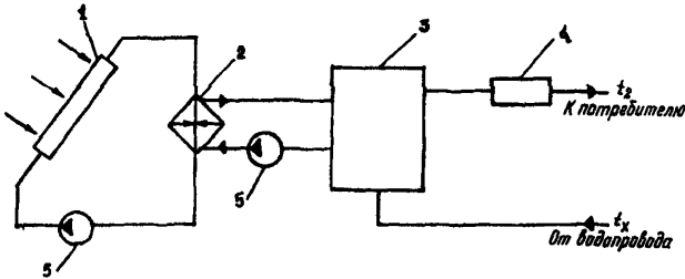
Рис.2. Принципиальная схема системы солнечного горячего водоснабжения
