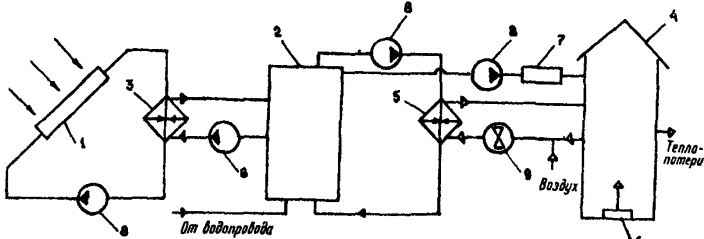
Рис.1. Принципиальная схема системы солнечного теплоснабжения
