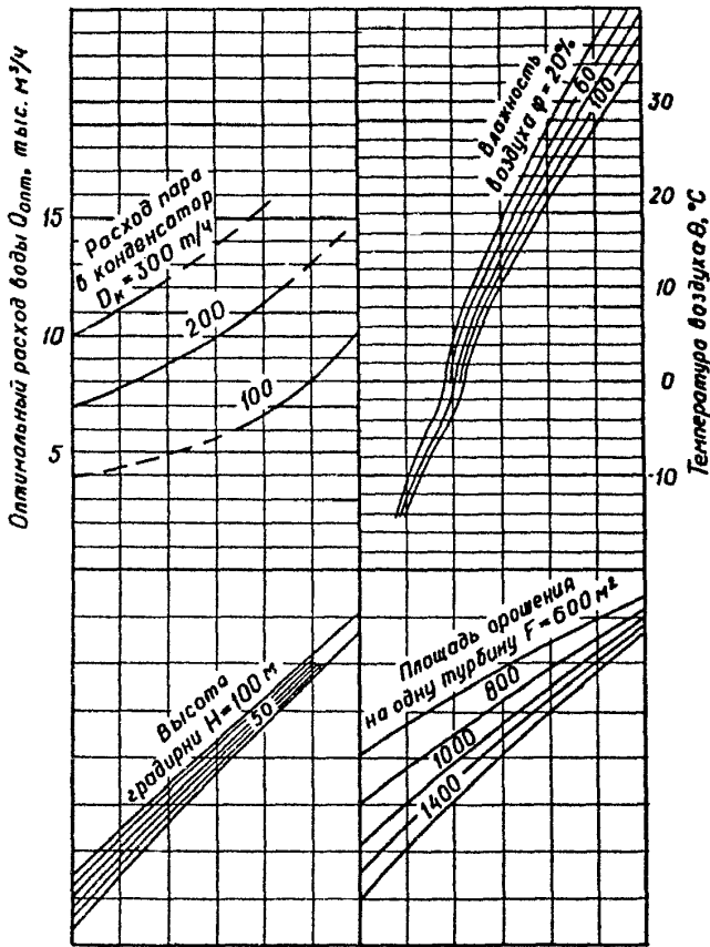
Рис. 6. Номограмма для определения оптимального расхода воды в конденсатор турбины ПТ-135/165-130/15
