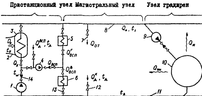
Рис. 3. Принципиальная схема оборотной системы водоснабжения
