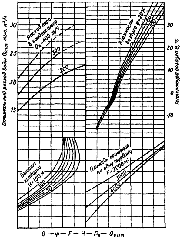
Рис. 9. Номограмма для определения оптимального расхода воды в конденсатор турбины К-203-130
