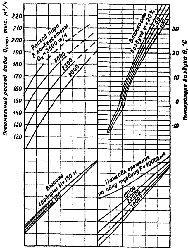
Рис. II. Номограмма для определения оптимального расхода воды в конденсаторы турбины К-1000-60/3000
