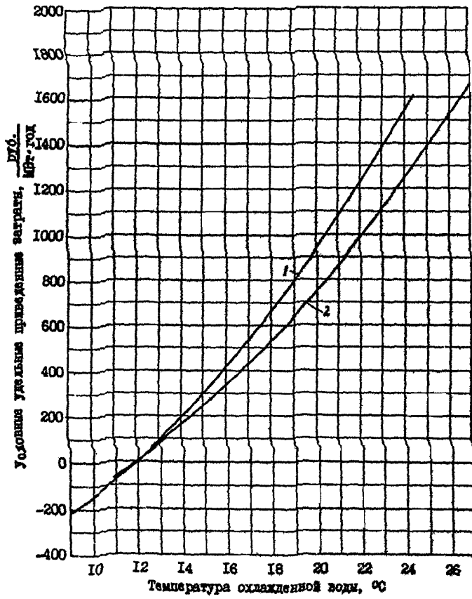
Рис. 2. График для определения условных удельных приведенных затрат по компенсации изменения оттока электроэнергии конденсационными турбинами на 1 МВт тепловой нагрузки градирей в зависимости от температуры охлаждающей воды:
