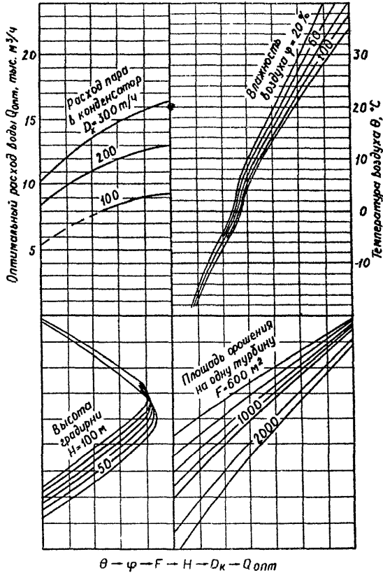
Рис. 5. Номограмма для определения оптимального расхода воды в конденсатор турбины Т-110/120-133-3
