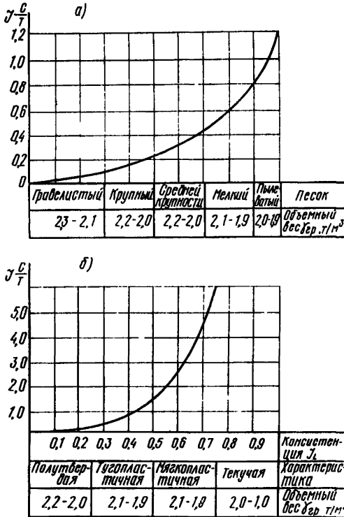
Рис. 2. График для выбора коэффициента l : а — песчаные грунты; б — глинистые грунты
