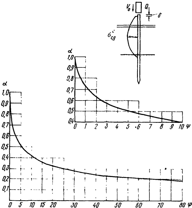
Рис. 1. График \alpha=f(\psi)
