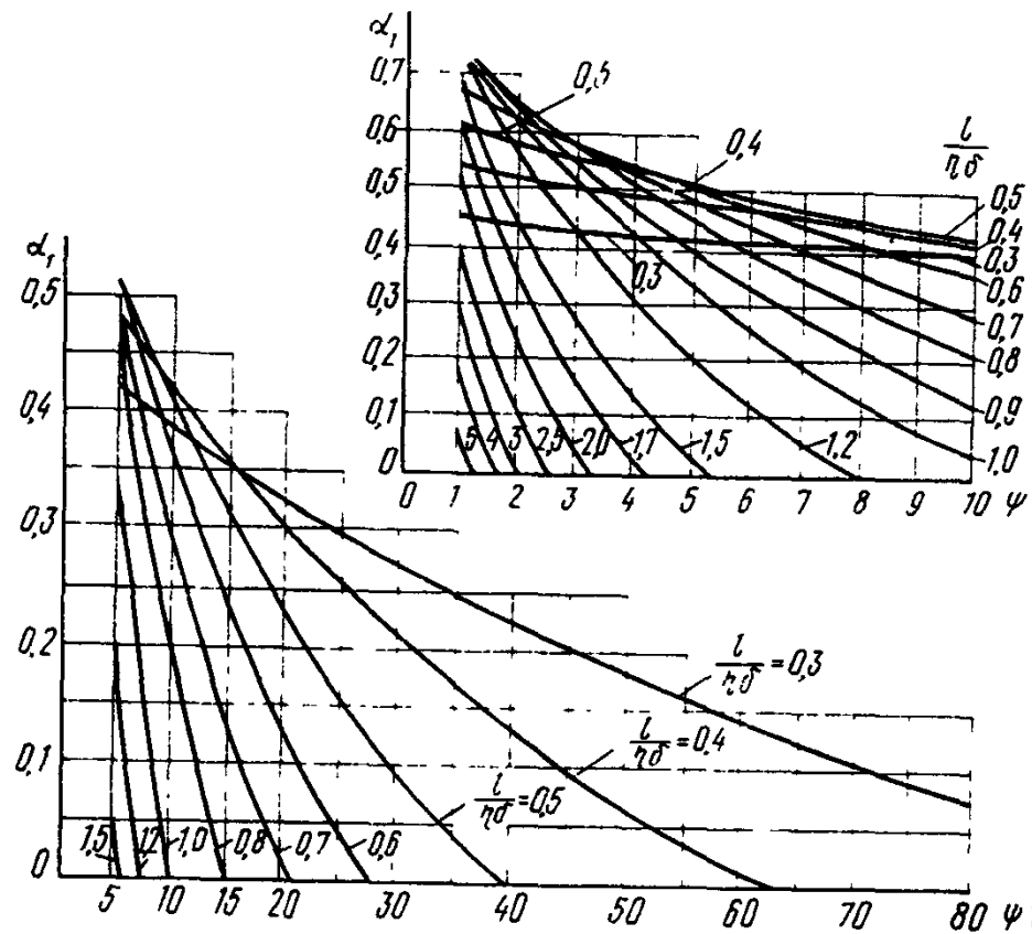
Рис. 4. Графики \alpha_1=f(\psi, l/\eta\delta)
