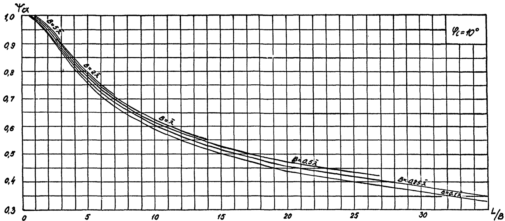
Рис. П. I. II. График для определения коэффициента \chi_c при угле \psi = 10^\circ .
