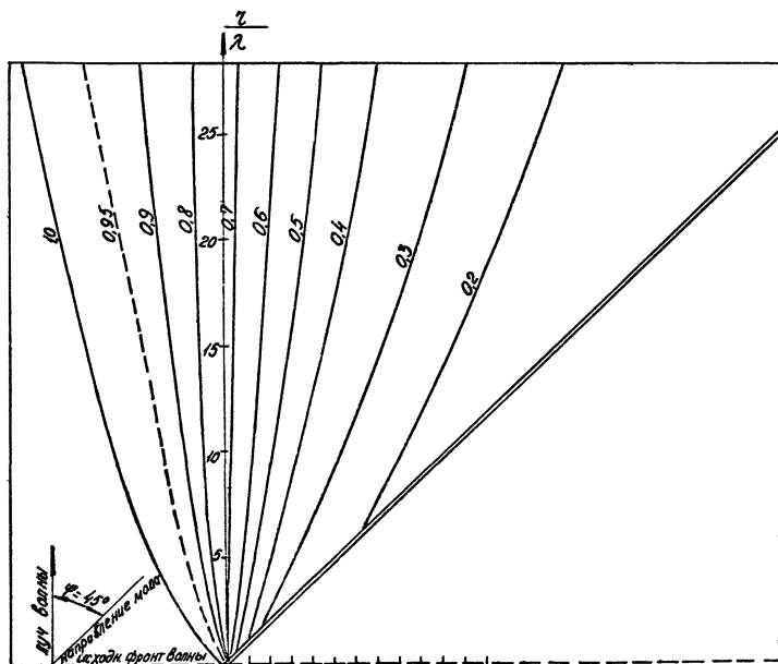
Рис. П. I. 6. График для определения коэффициента дифракции k_{dif,s} для угла \psi = 45^\circ .
