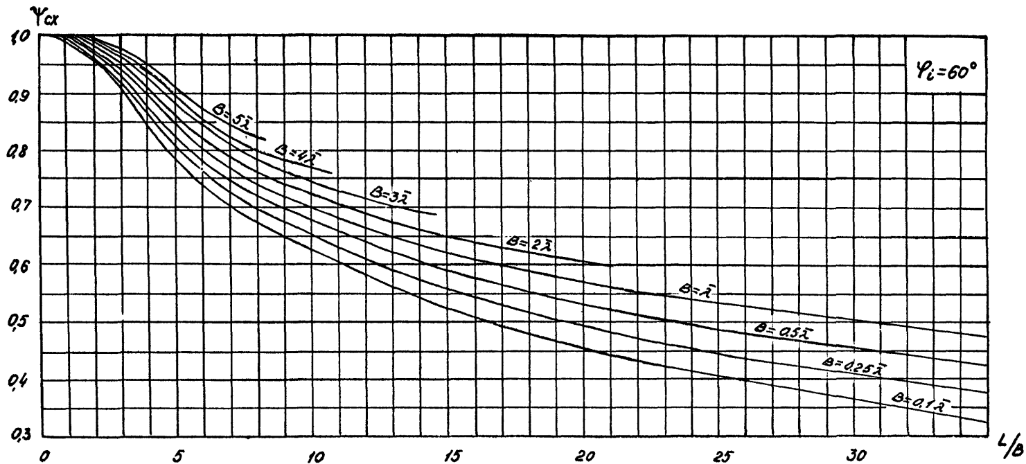
Рис. П.І.ІБ. График для определения коэффициента \gamma_c при угле \psi = 60^\circ .
