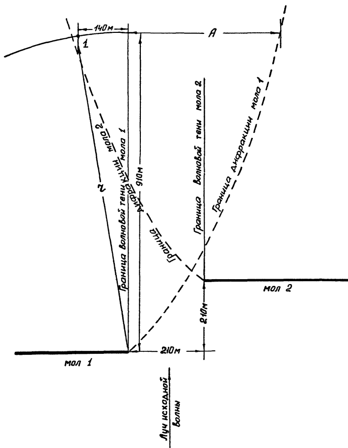
Рис. П.2.3. Схема к примеру расчета коэффициента дифракции на акватории, огражденной сходящимися молами.
