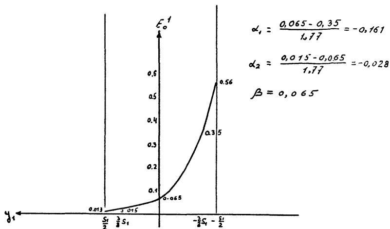
Рис. П.2.8. Схема распределения начальной энергии на фронте S_1 , к примеру расчета коэффициента дифракции на акватории, огражденной перекрывающимися молами.
