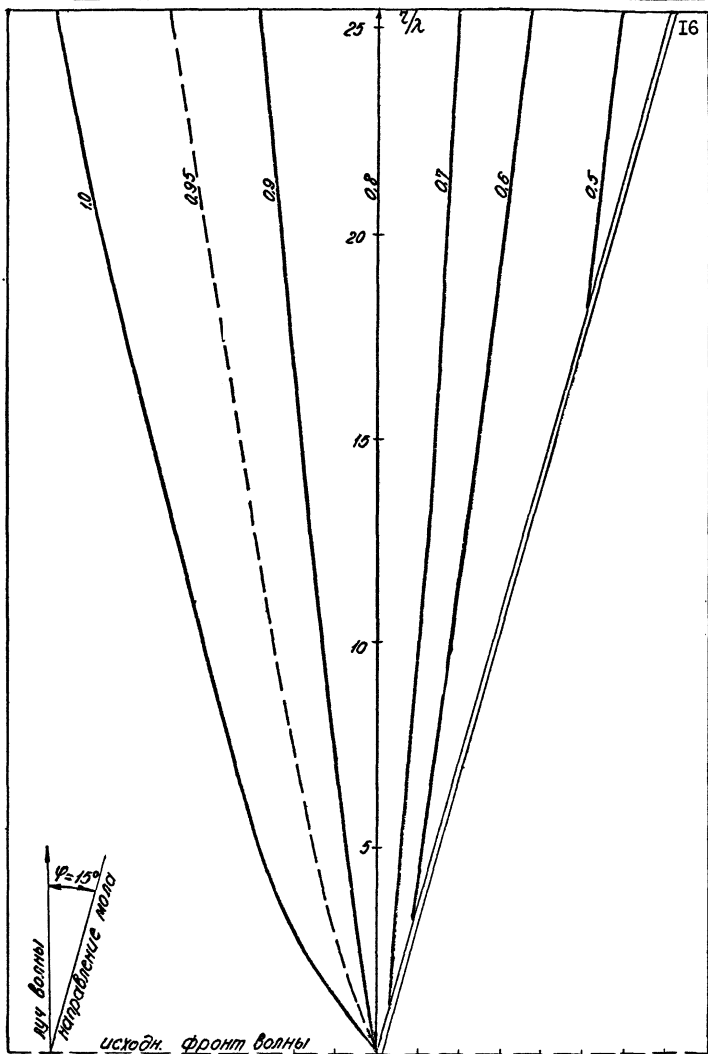
Рис. П.Г.3. График для определения коэффициента дифракции k_{dif,s} для угла \varphi = 15^\circ .
