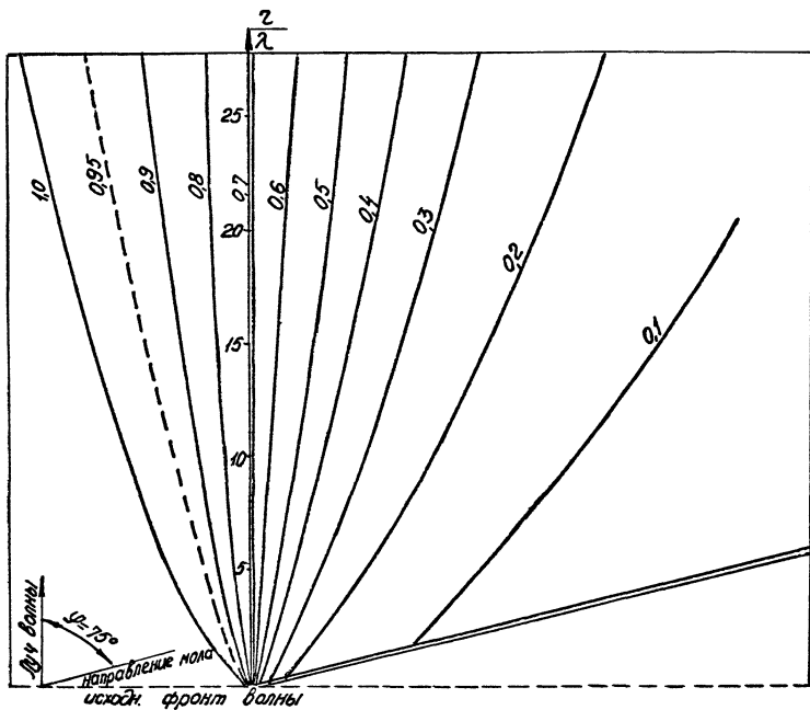
Рис. П.1.8. График для определения коэффициента дифракции k_{dif,s} для угла \psi = 75^\circ .
