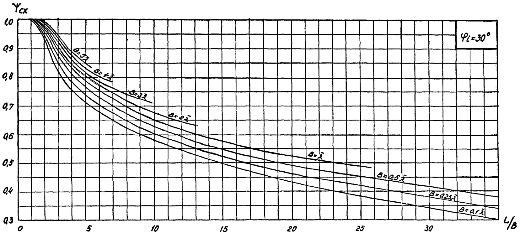
Рис. П.Г.ИИ. График для определения коэффициента \gamma_{сх} при угле \varphi = 30^\circ .
