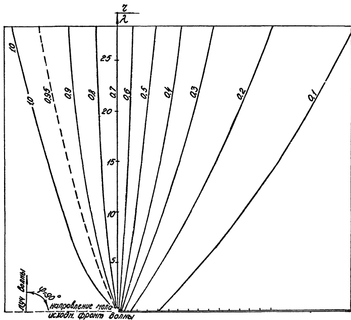
Рис. П.1.9. График для определения коэффициента дифракции k_{dif,s} для \psi = 90^\circ .
