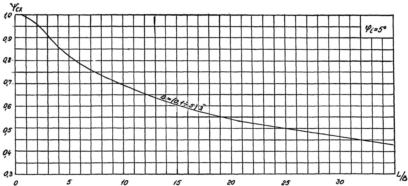
Рис. П. I. IO. График для определения коэффициента \psi_{сх} при угле \psi = 5^\circ .
