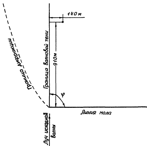
Рис П.2.1 . Схема к примеру расчета коэффициентов дифракции на акватории, огражденной одиночным прямолинейным молотом.
