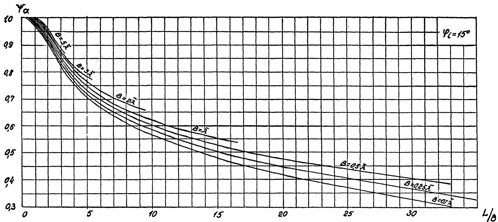
Рис. П.І.12. График для определения коэффициента \psi_c при угле \psi = 15^\circ .
