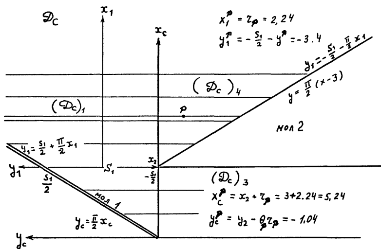
Рис. П.2.7. Схема расчетной области D_c к примеру расчета коэффициента дифракции на акватории, огражденной перекрывающимися молами.
