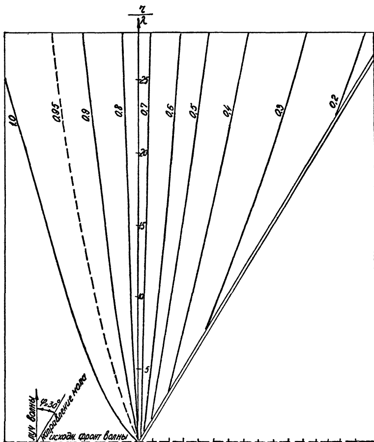
Рис. П. I. 5. График для определения коэффициента дифракции k_{difs} для угла \varphi = 30^\circ .
