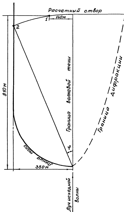
Рис. П.2.2. Схема к примеру расчету коэффициентов дифракции на акватории, огражденной одиночным криволинейным в плане молом.
