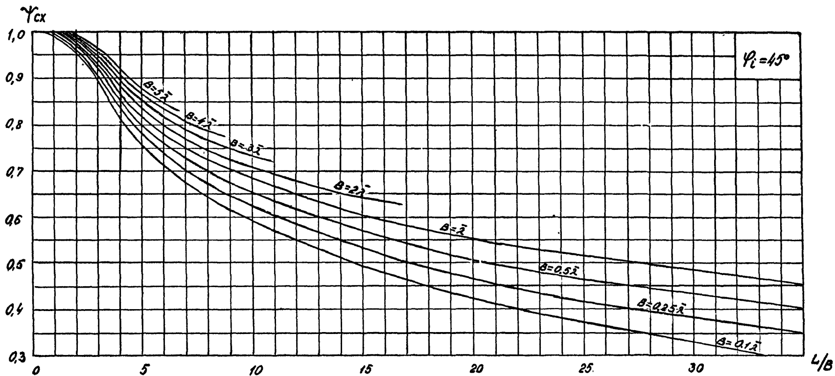
Рис. П.1.15. График для определения коэффициента \gamma_c при угле \varphi = 45^\circ .
