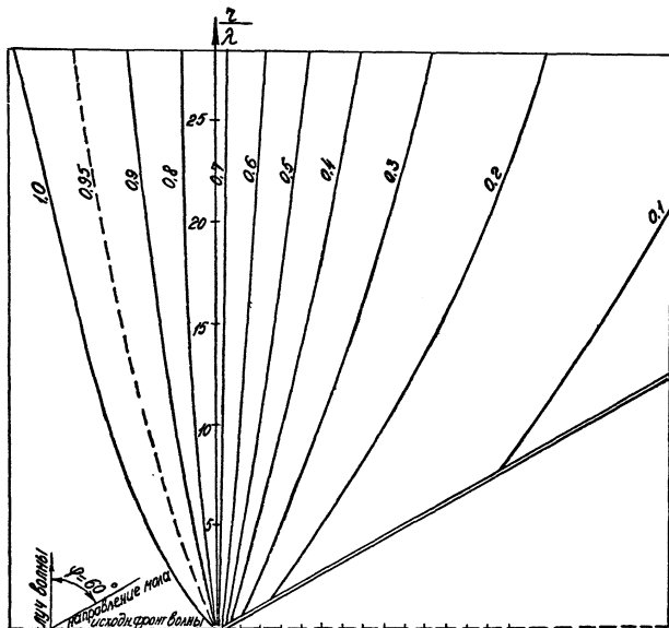
Рис. П.1.7. График для определения коэффициента дифракции k_{difs} для \psi = 60^\circ .
