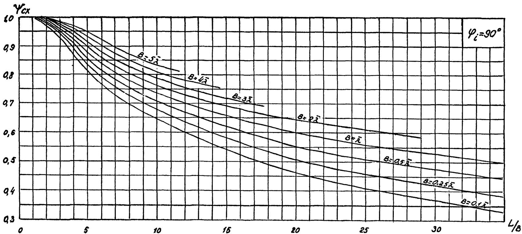
Рис. П. I. 18. График для определения коэффициента \Psi_c при угле \varphi = 90^\circ .
