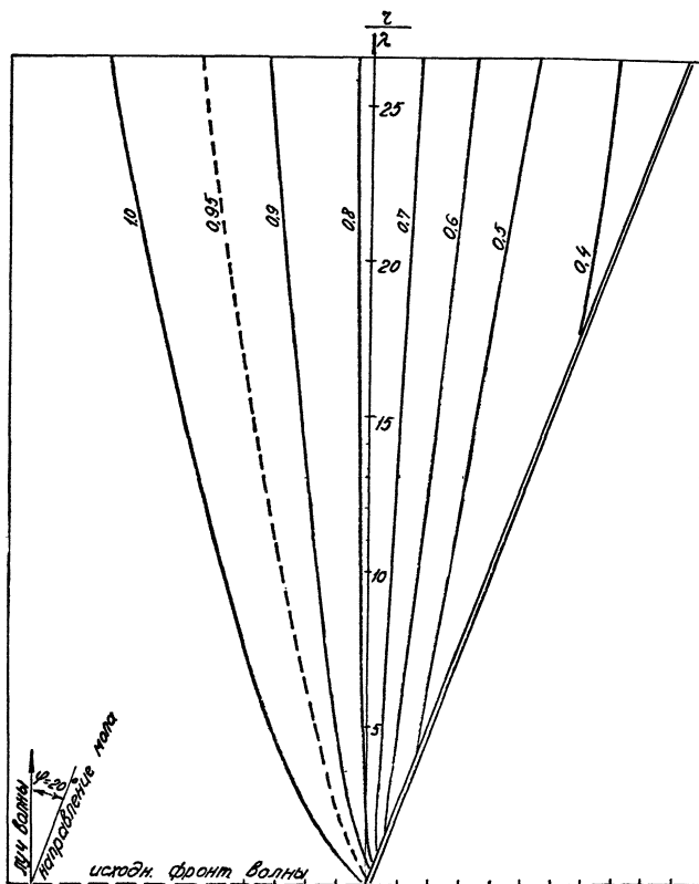
Рис П.1.4. График для определения коэффициента дифракции k_{dif,s} для \psi = 20^\circ .
