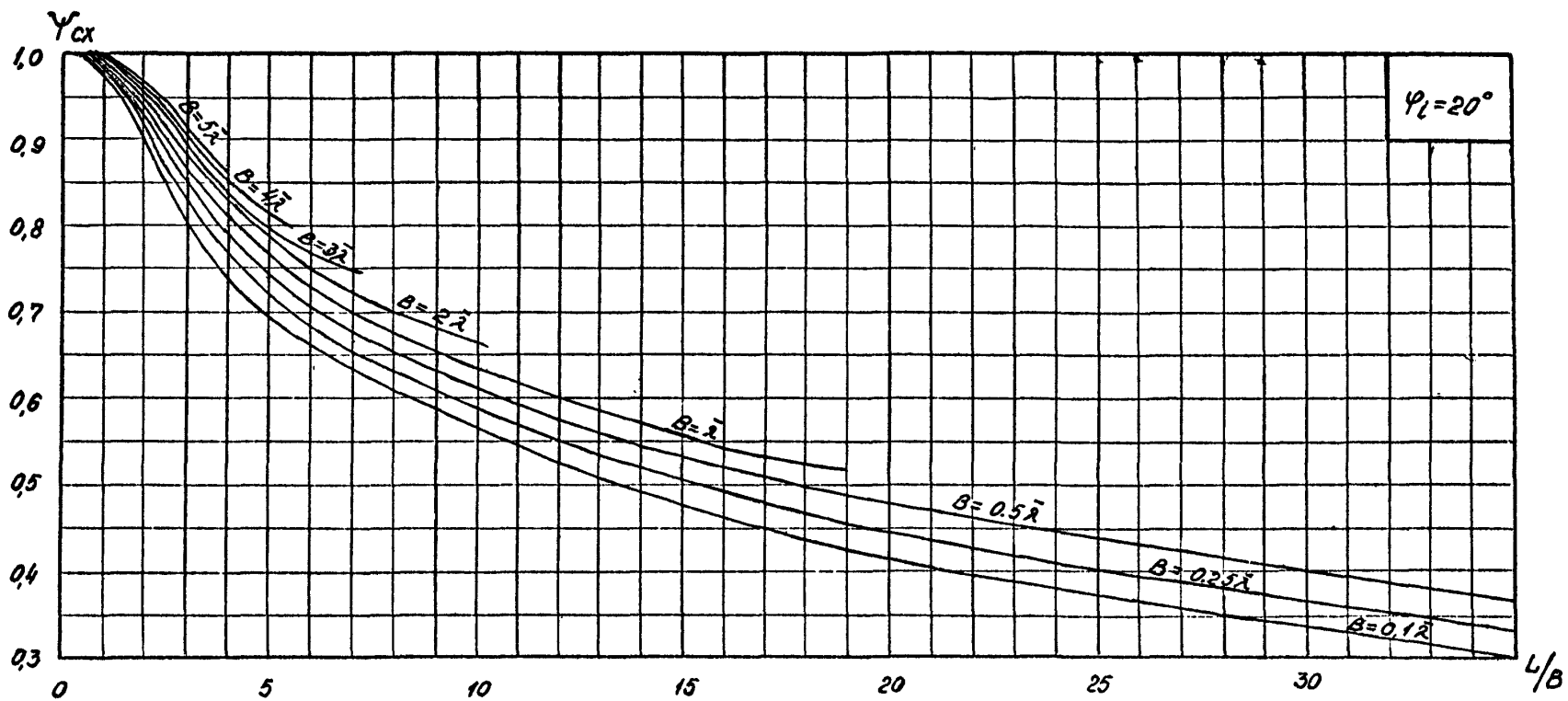
Рис. П. 1.13. График для определения коэффициента \psi_c при угле \psi = 20^\circ .
