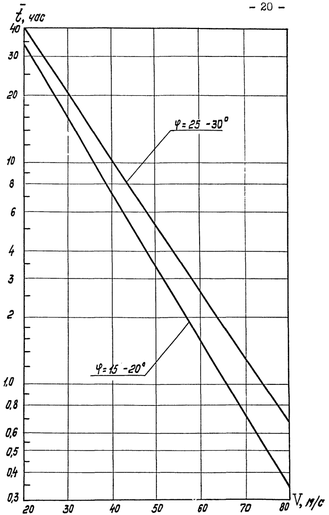
Рис. 3. Номограмма для определения средней продолжительности непрерывного действия расчетных скоростей ветра для широт 15 - 20° и 25 - 30°.
