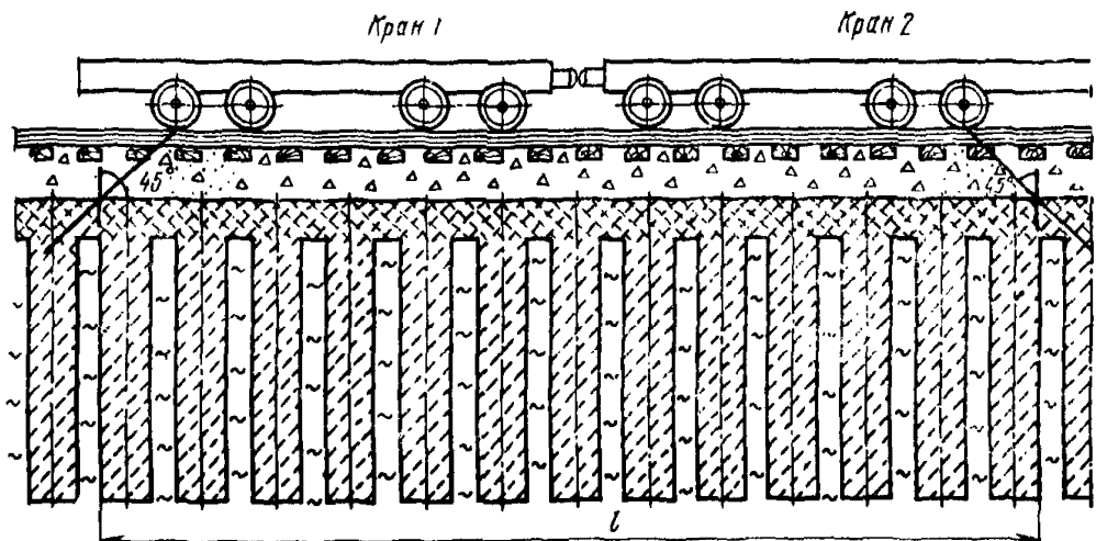
Рис. 5. Схема расчетного элемента основания подкрановых путей
