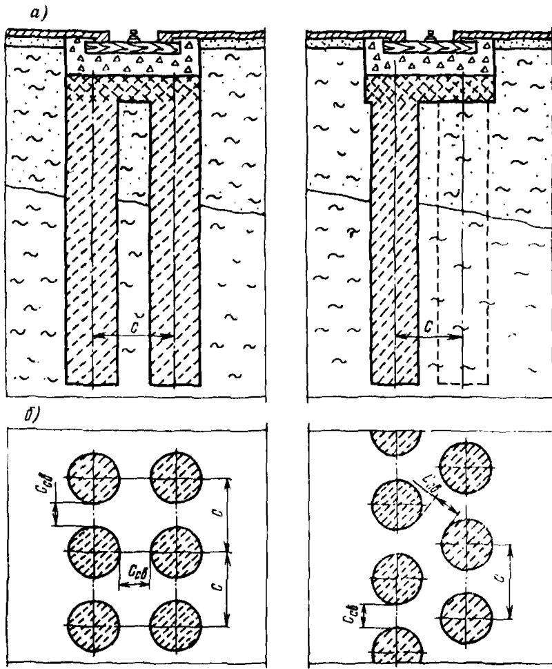
Рис. 4. Схемы подкрановых путей на илоцементных сваях (слева — без относительного смещения свай в рядах, справа — с относительным смещением свай в рядах): а — поперечный разрез; б — план
