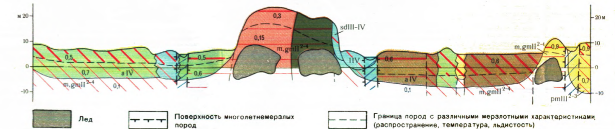
ИНЖЕНЕРНО-ГЕОКРИОЛОГИЧЕСКИЙ РАЗРЕЗ ПО ЛИНИИ I-I' И МАКЕТУ II
