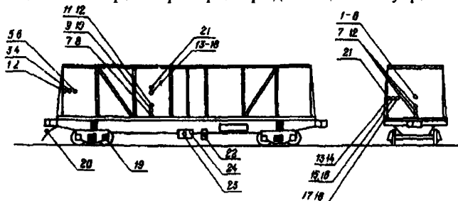
Рис.5. Расположение датчиков (1-24) на контрольном вагоне
