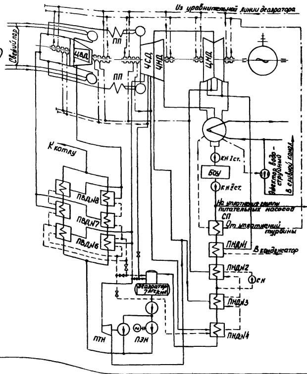
Принципиальная тепловая схема
