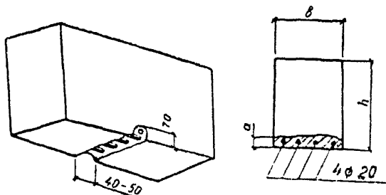
Рисунок 3 – Продольная арматура в середине пролета
