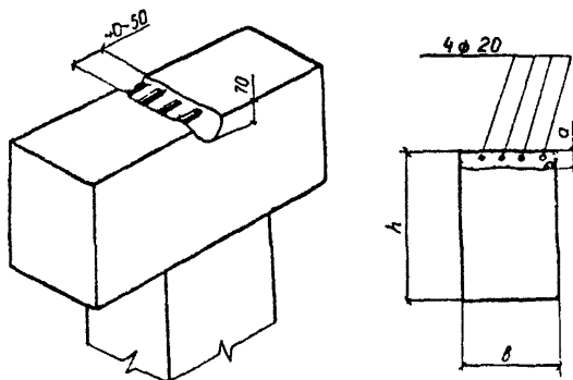
Рисунок 4 – Продольная арматура над опорой
