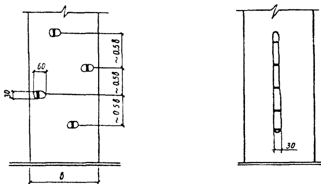
Рисунок 7 – Вскрытие хомутов путем пробивки вертикальной борозды на боковой грани колонны
