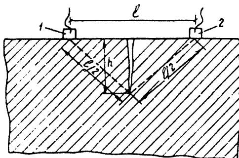
1 – излучатель; 2 – приемник
