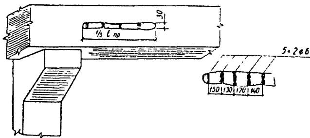
Рисунок 5 – Поперечная арматура у опор
