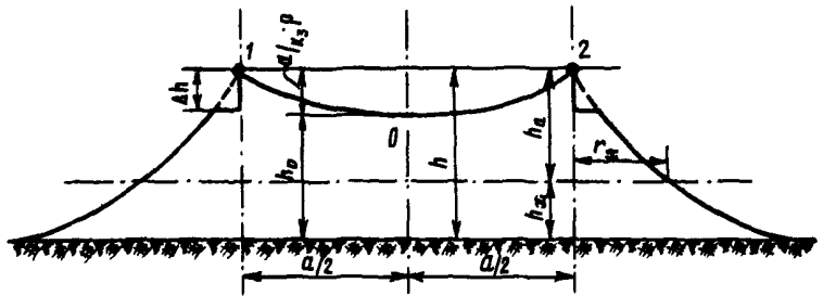
Рис.18. Зона защиты двух тросовых молниезащитов высотой более 30 м
