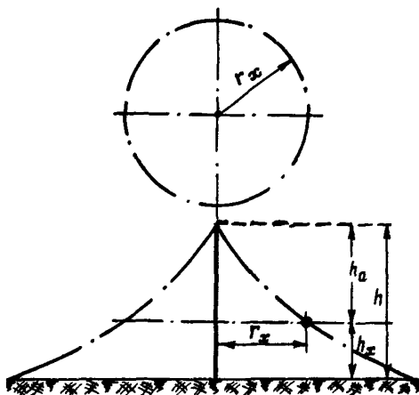
Рис.1. Зона защиты одиночного стержневого молниеотвода высотой до 60 м:
