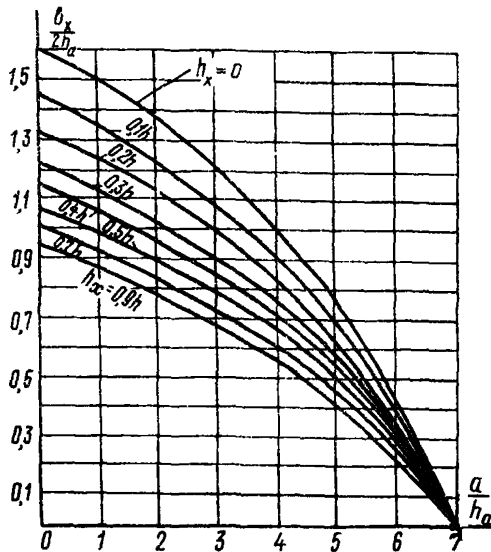
Рис.8. Значения наименьшей ширины зоны защиты \delta_x двух стержневых молниеотводов высотой h \leq 30 м для \frac{a}{h_a} = 0+7
