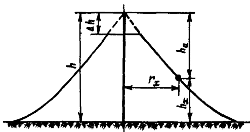
Рис.2. Зона защиты одиночного стержневого молниеотвода высотой более 60 м:
