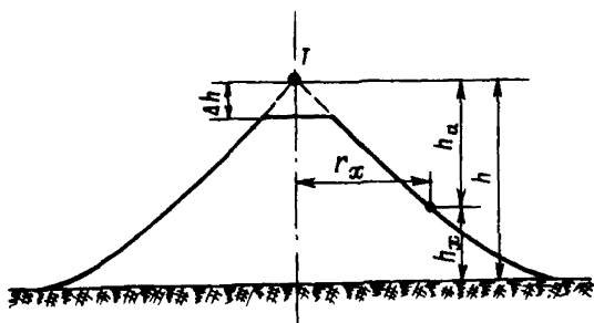
Рис.14. Зона защиты одиночного тросового молниествода высотой более 30 м
