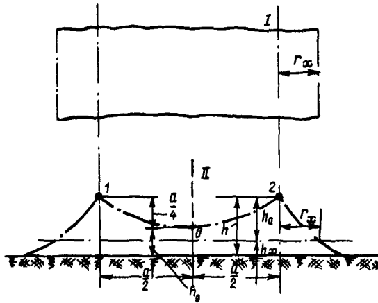
Рис.17. Зона защиты двух тросовых молниезащитов I и 2 высотой до 30 м:
