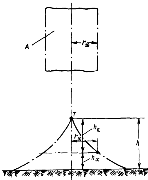
Рис.13. Зона защиты одиночного тросового молниествода высотой до 30 м:
