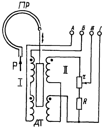
Рис.2. Принципиальная электрическая схема прибора модели 22364:
