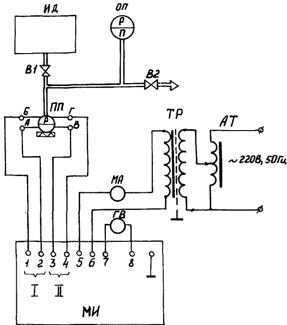
Рис.3. Схема соединений при проверке прибора с помощью магазина комплексной взаимной индуктивности;
